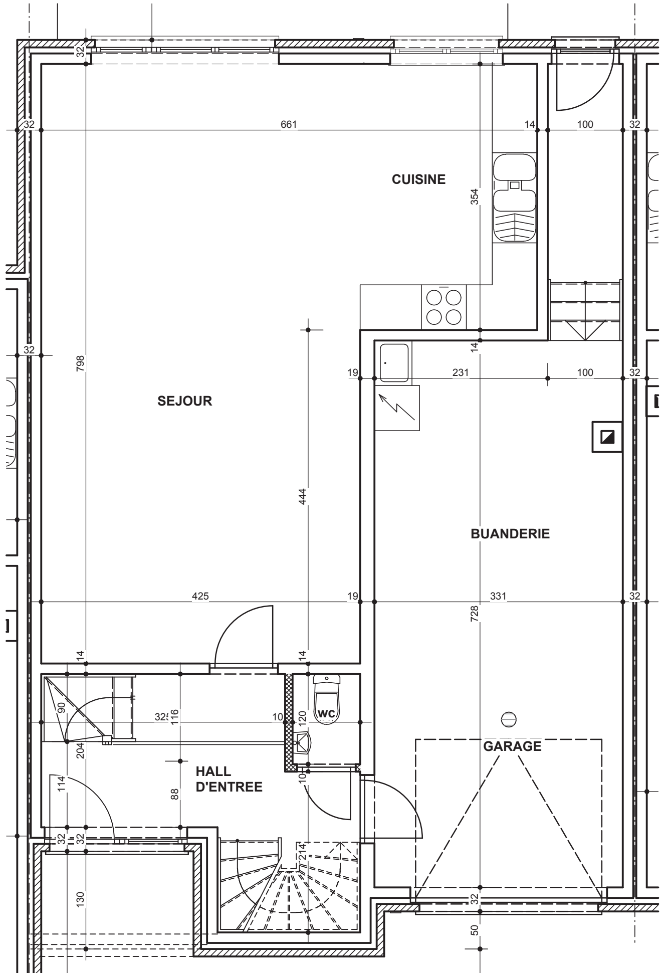
Maison 16b : Rez de chaussée
