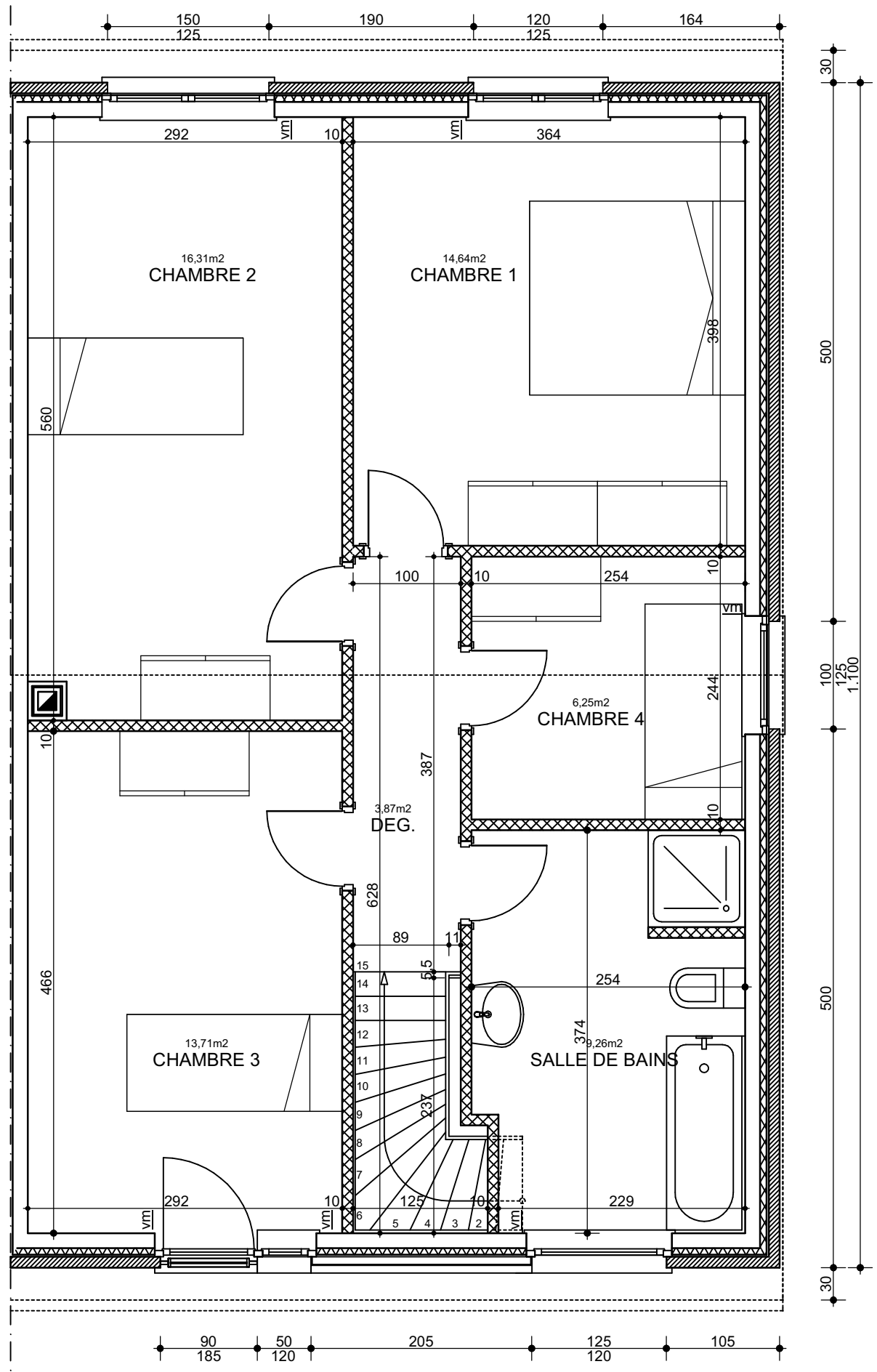
Awans : étage 1 maison 7
