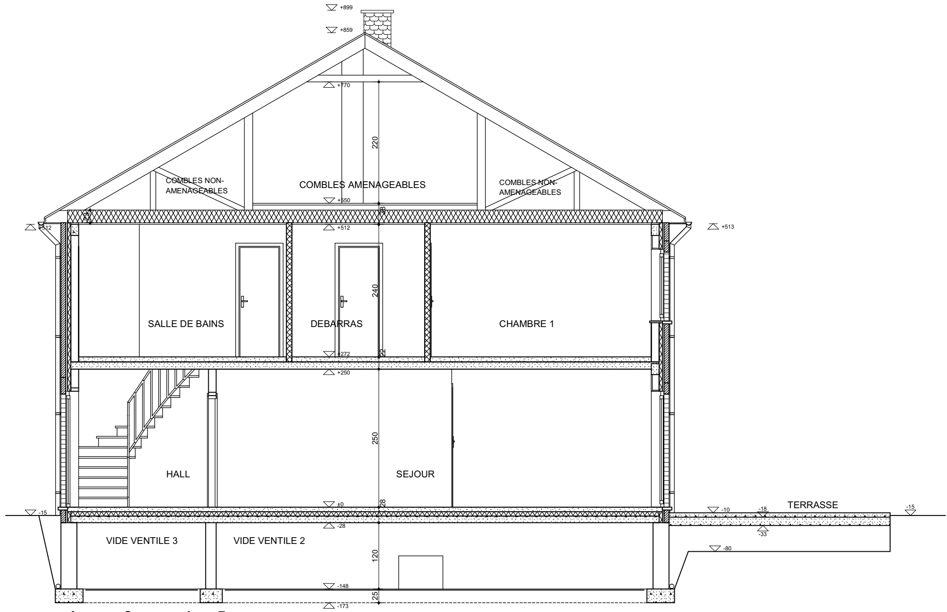
Awans : Coupe maison 7
