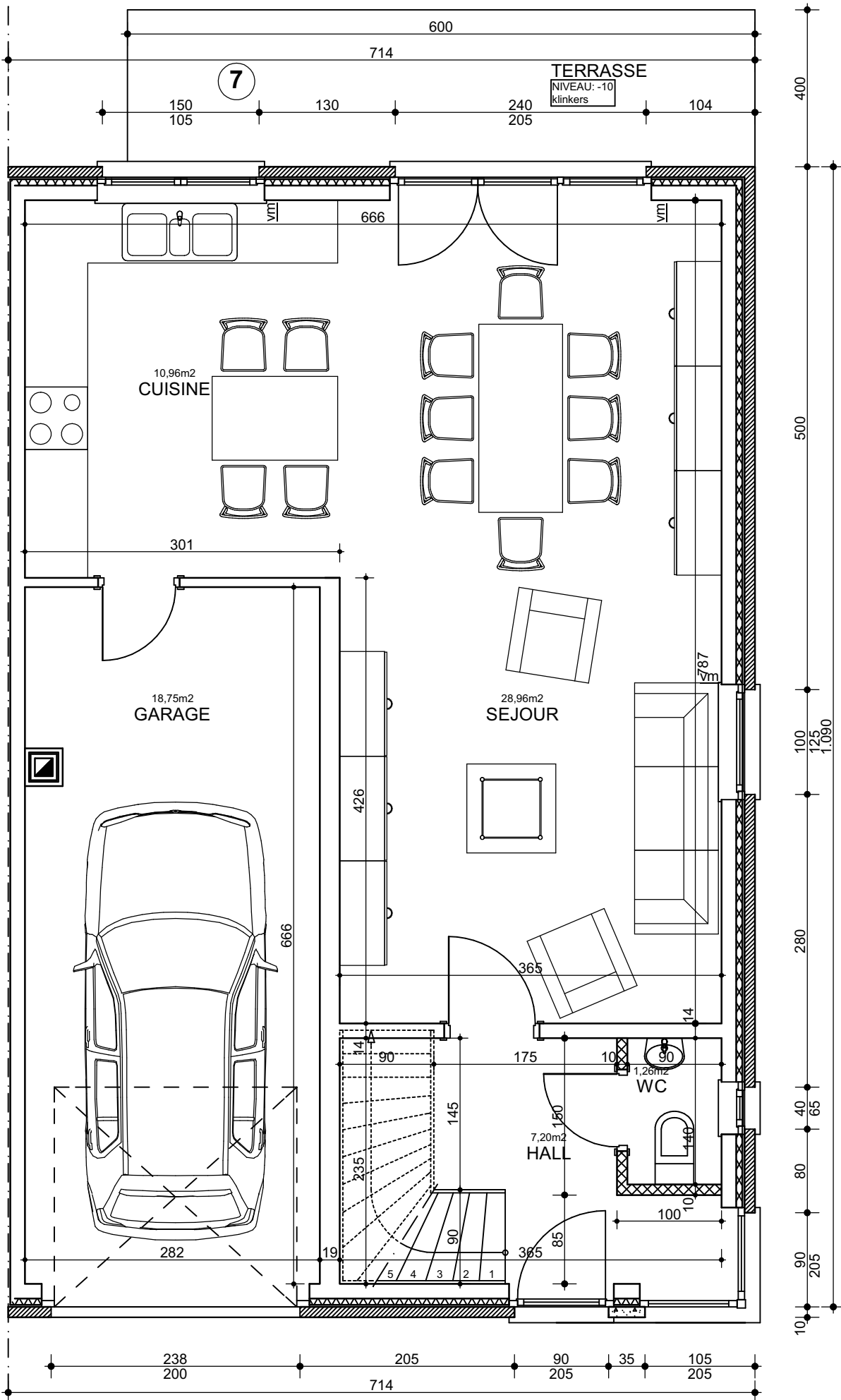
Awans : rez-de-chaussée maison 7
