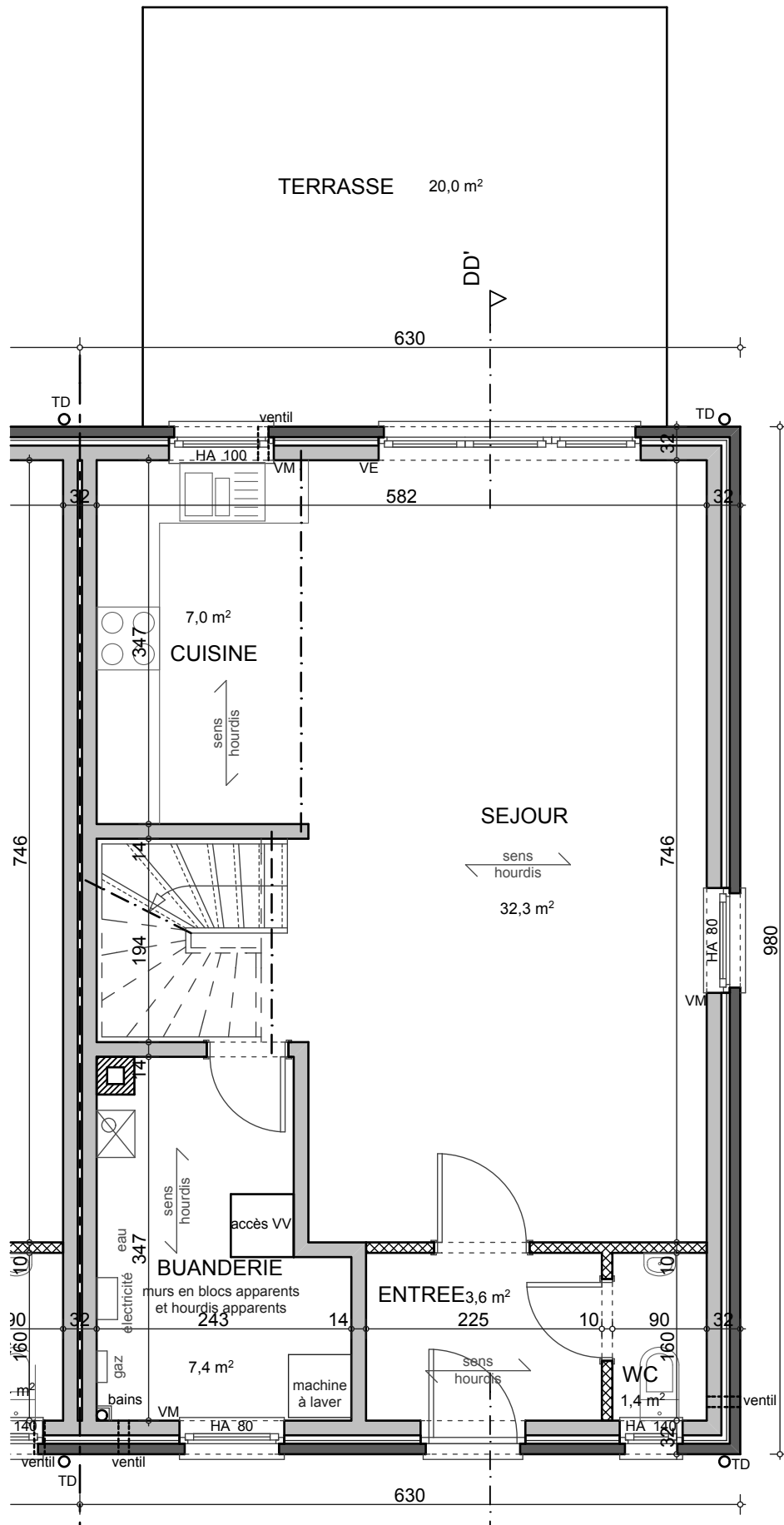
VIVEGNIS - rue d'Abooz MAISON 40B - REZ-DE-CHAUSSEE
