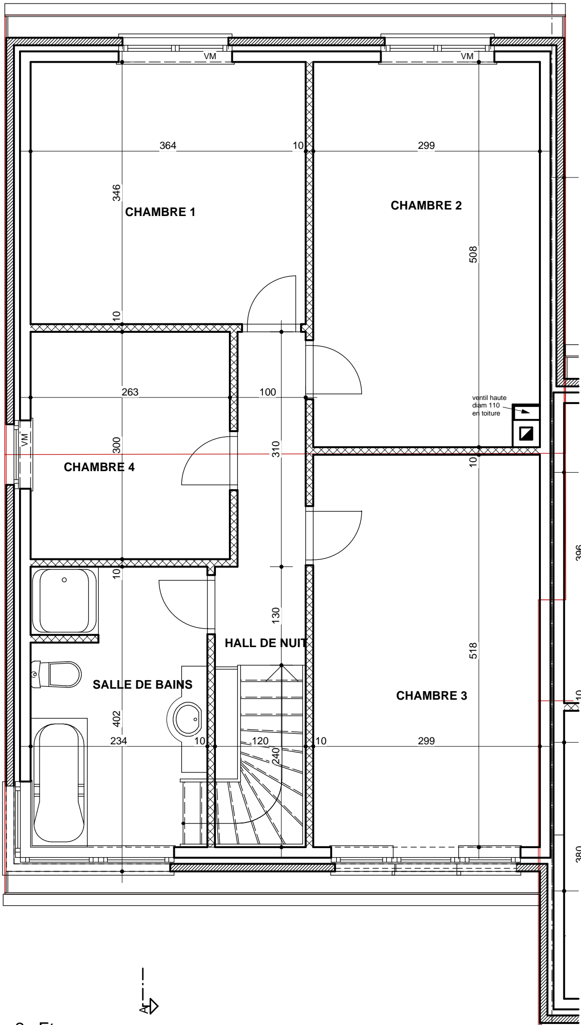
Maison 2 : Etage
