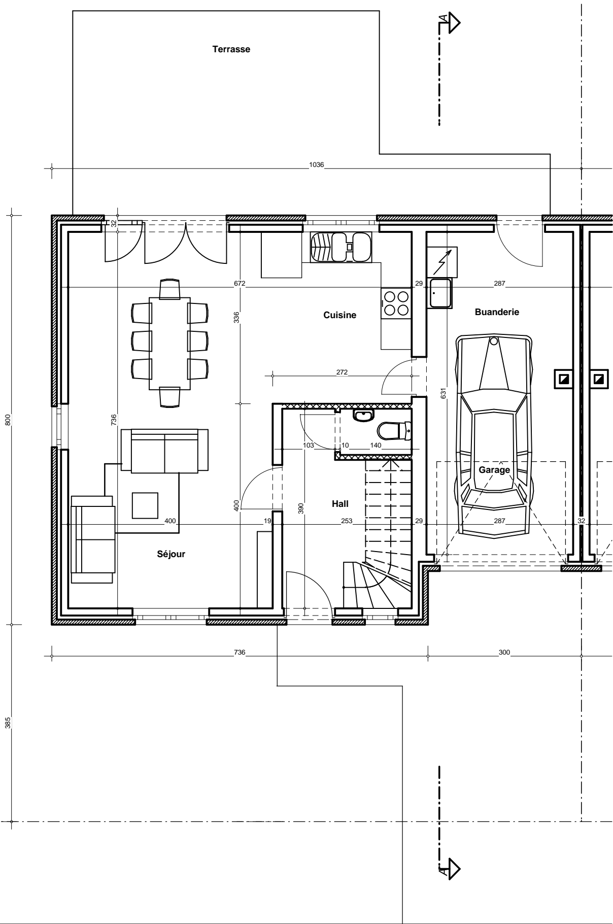
Maison 16 : Rez de Chaussée
