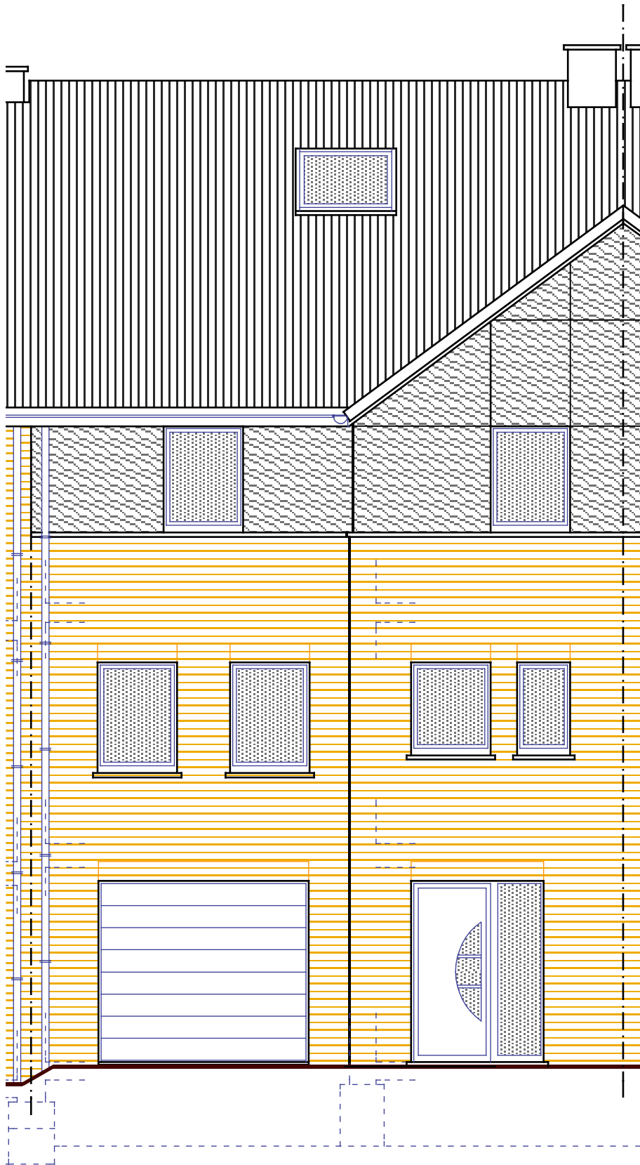
rue Grande Bruyère MAISON 5 - FACADE A RUE
