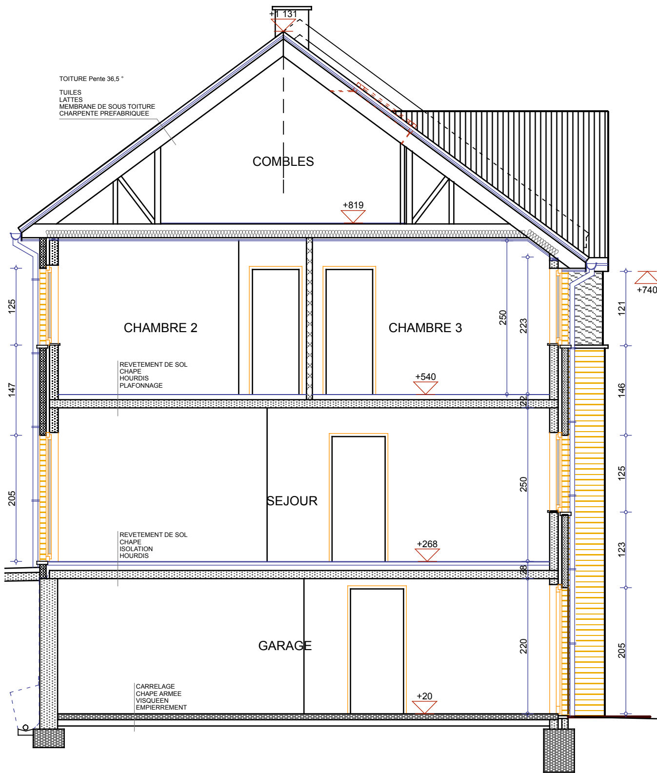
rue Grande Bruyère MAISON 5 - COUPE
