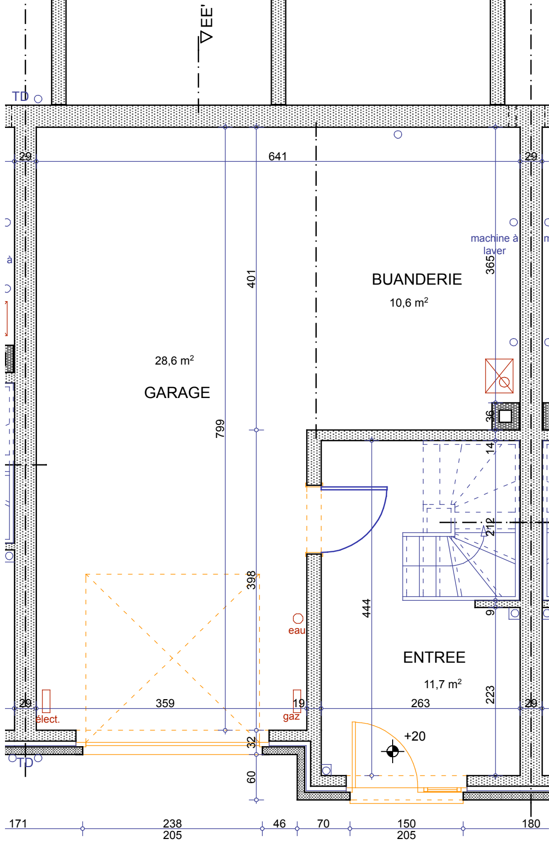
rue Grande Bruyère MAISON 5 - PLAN SOUS-SOL
