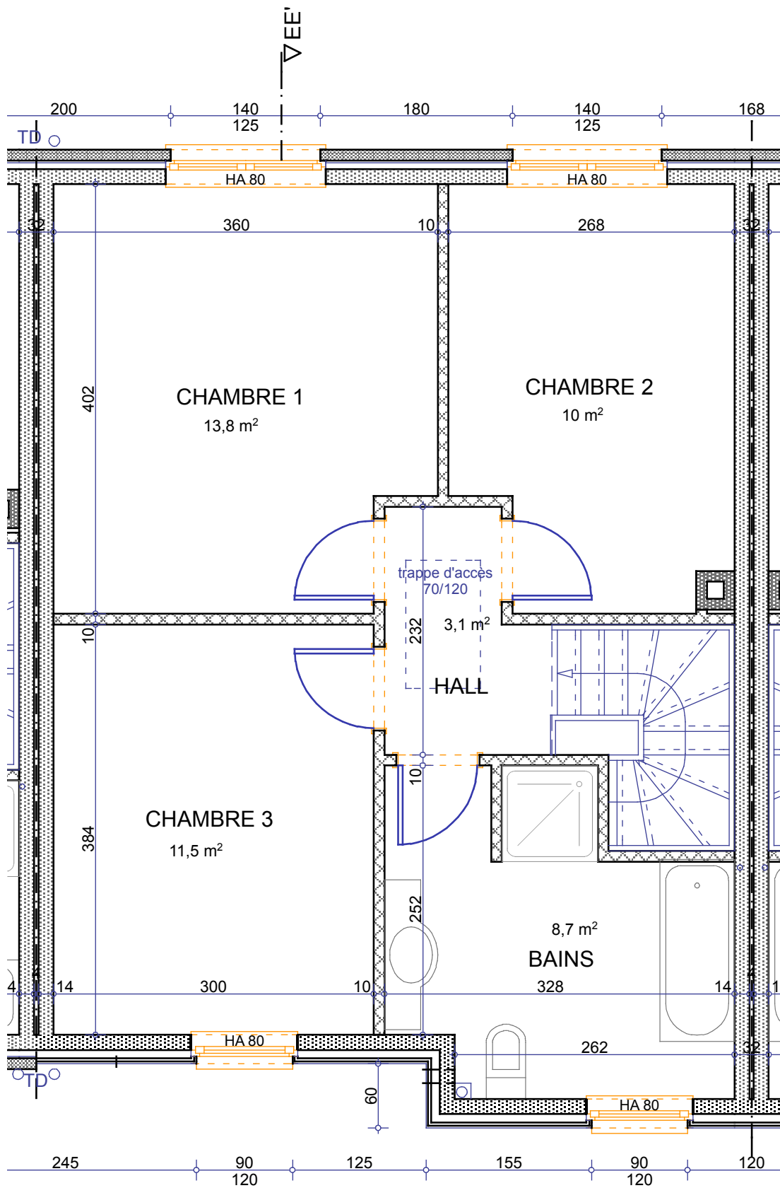
rue Grande Bruyère MAISON 5 - PLAN ETAGE
