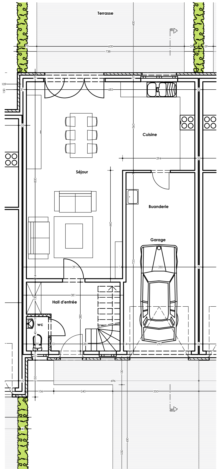
Maison 2 : Plan Rez-de-chaussée
