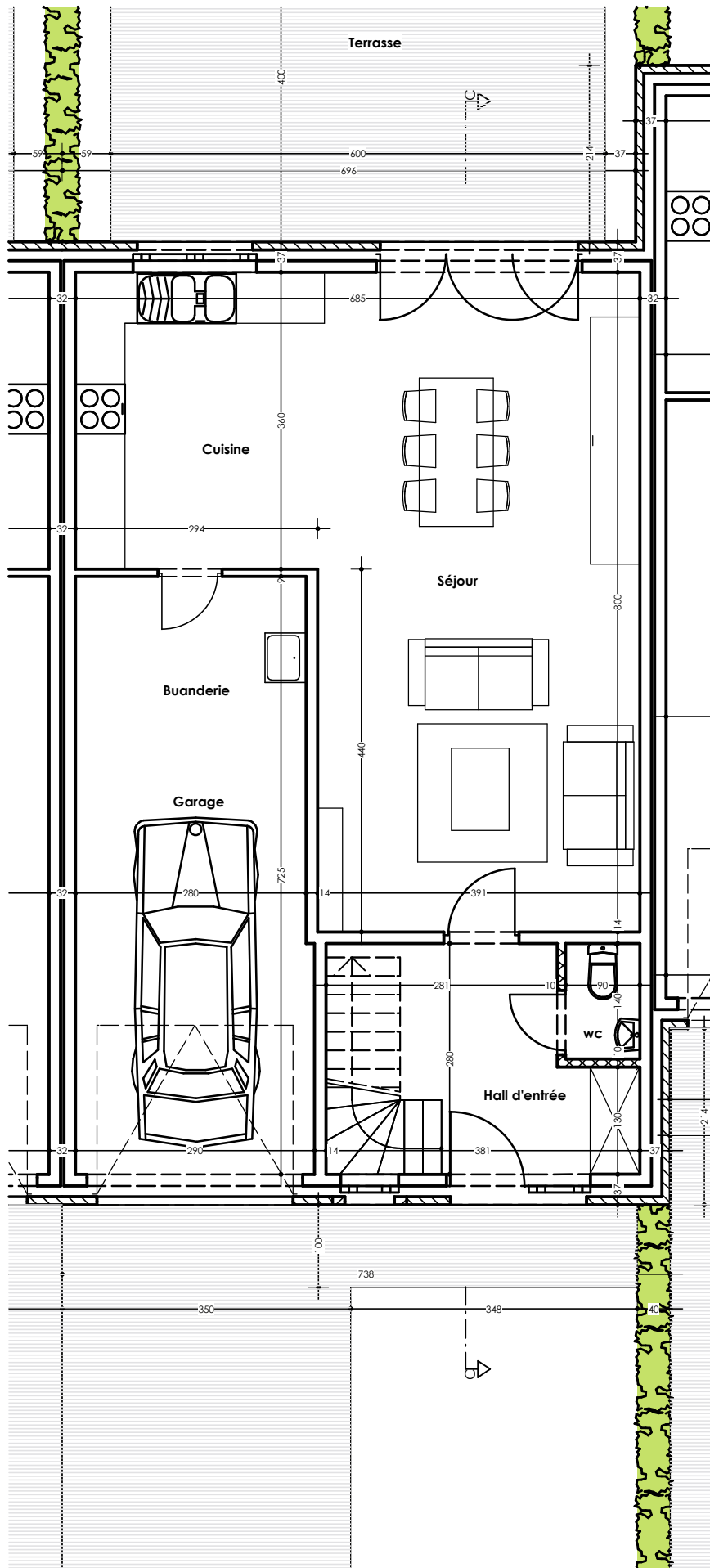
Maison 3 : Plan Rez-de-chaussée
