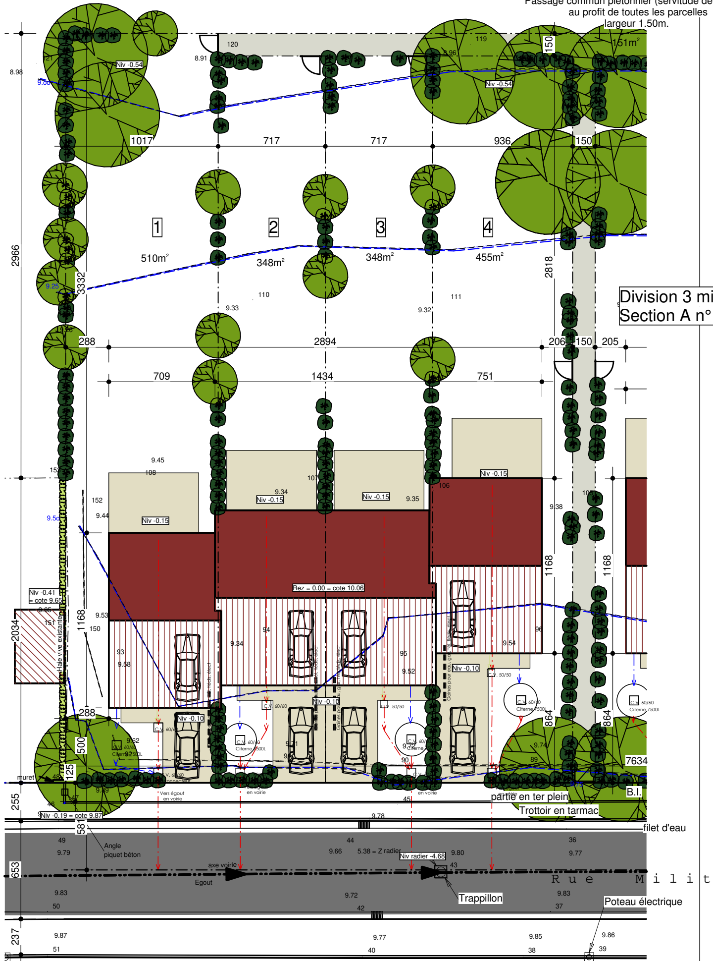
Plan d'implantation
