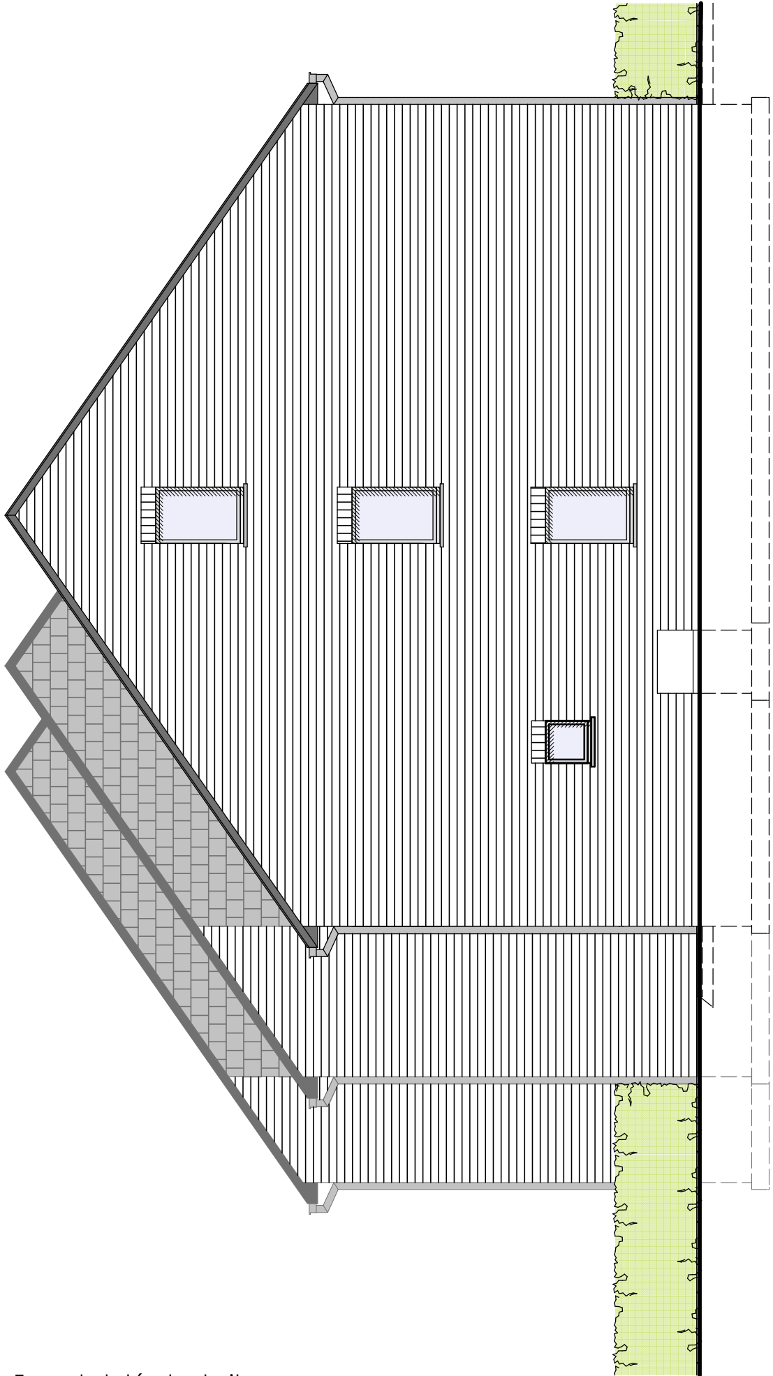
Maison 4 : Façade latérale droite
