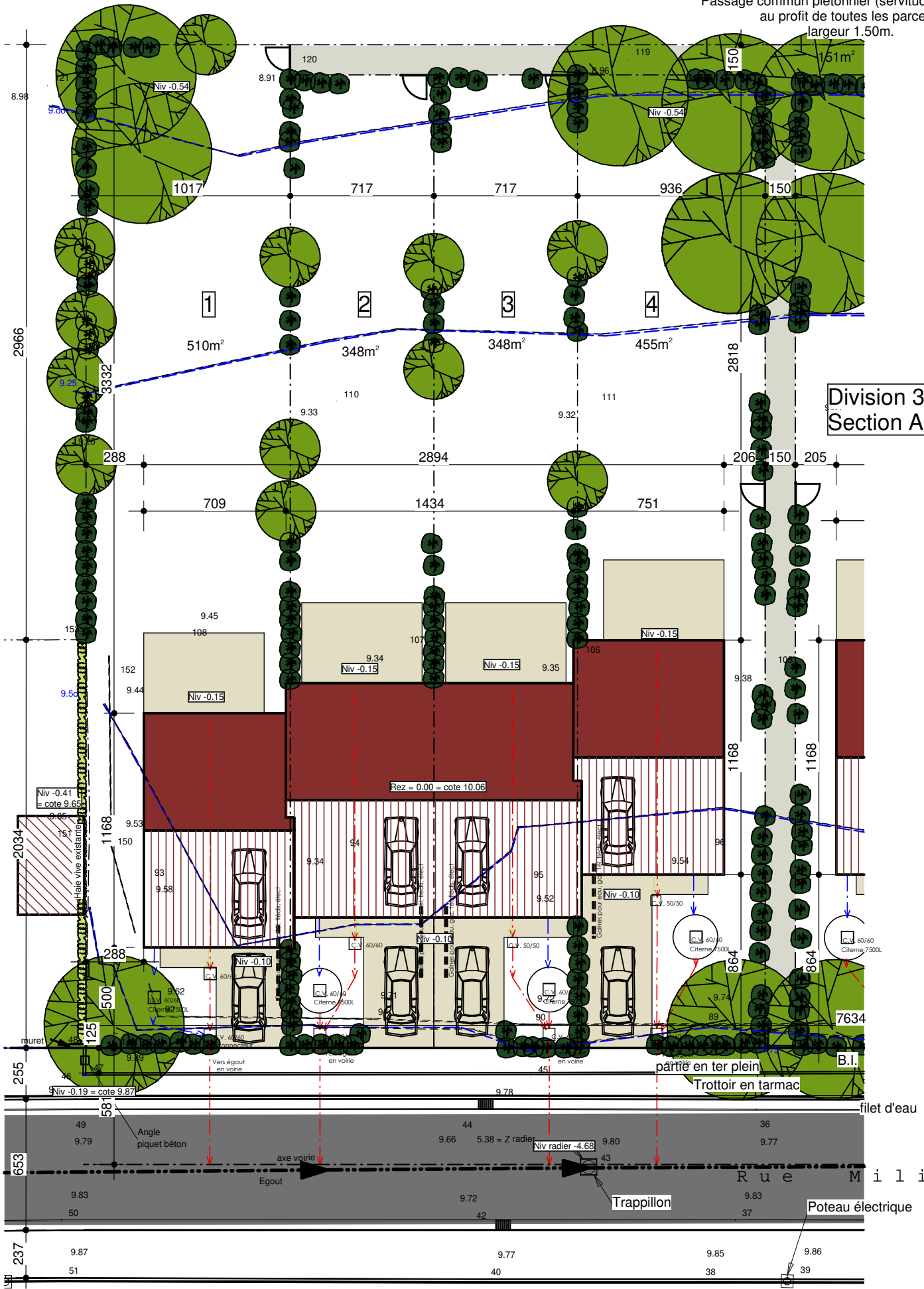
Plan d'implantation
