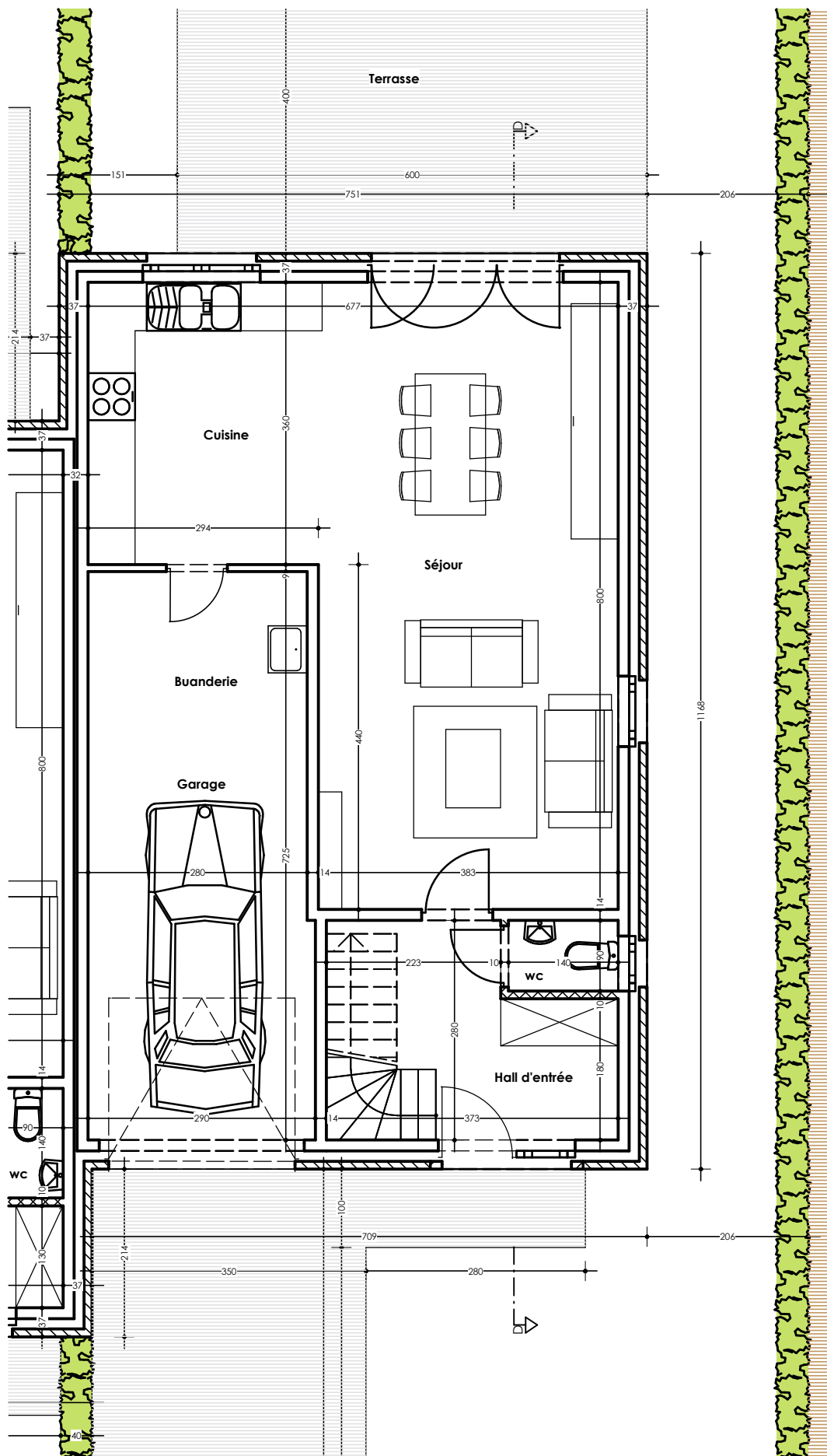
Maison 4 : Plan Rez-de-chaussée
