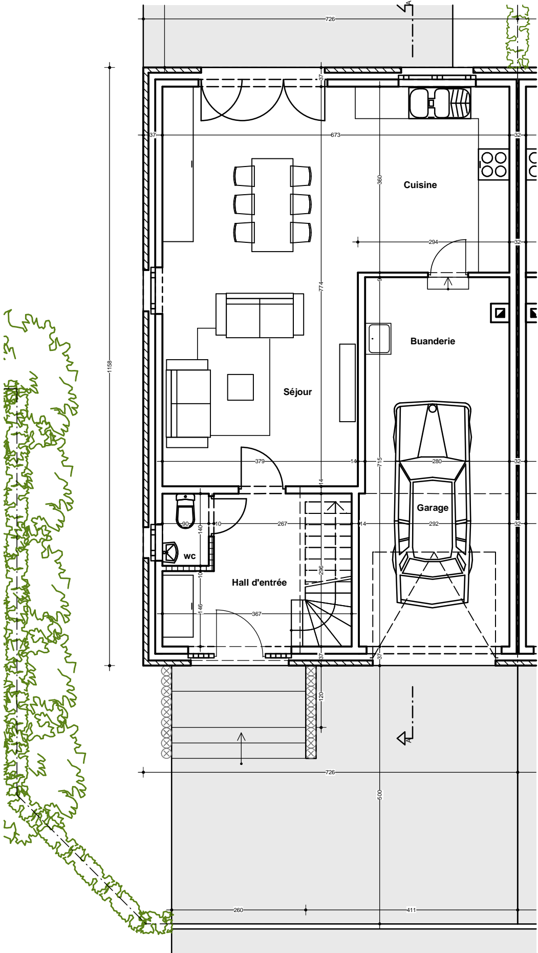
Maison 14 : Rez-de-chaussée
