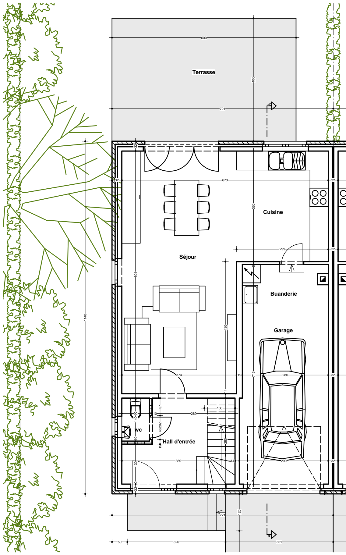
Maison 16 : Rez-de-chaussée
