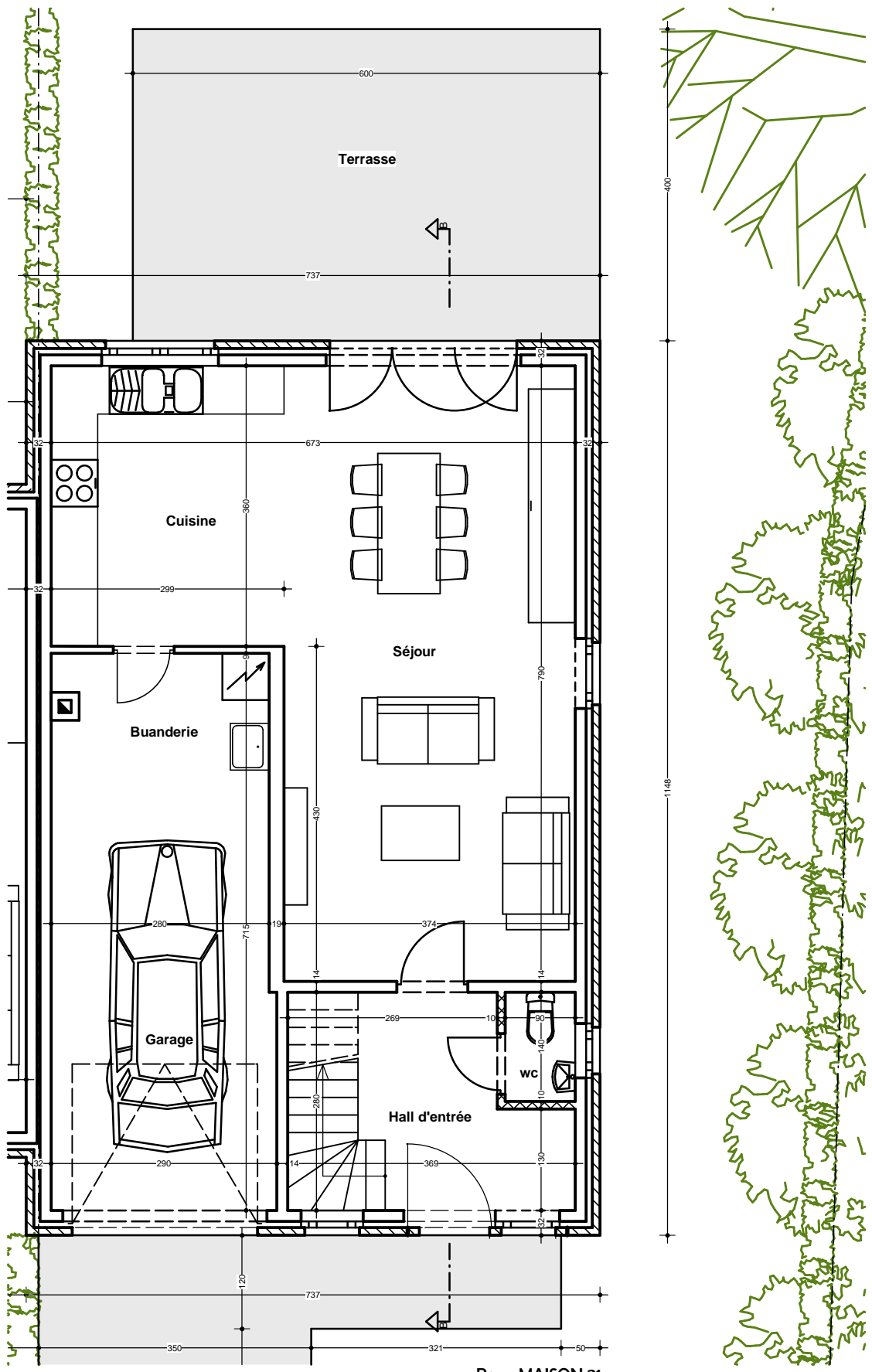
Rez - MAISON 21
