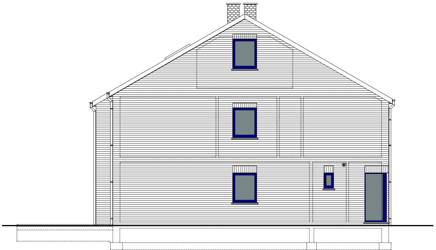
Baelen : Face latérale gauche maison 20
