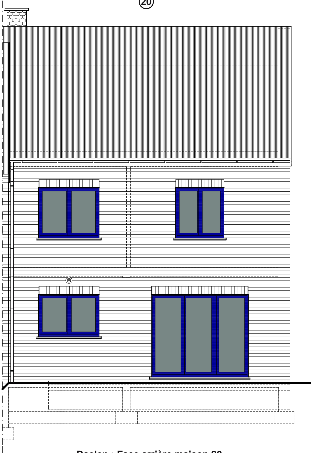
Baelen : Face arrière maison 20
