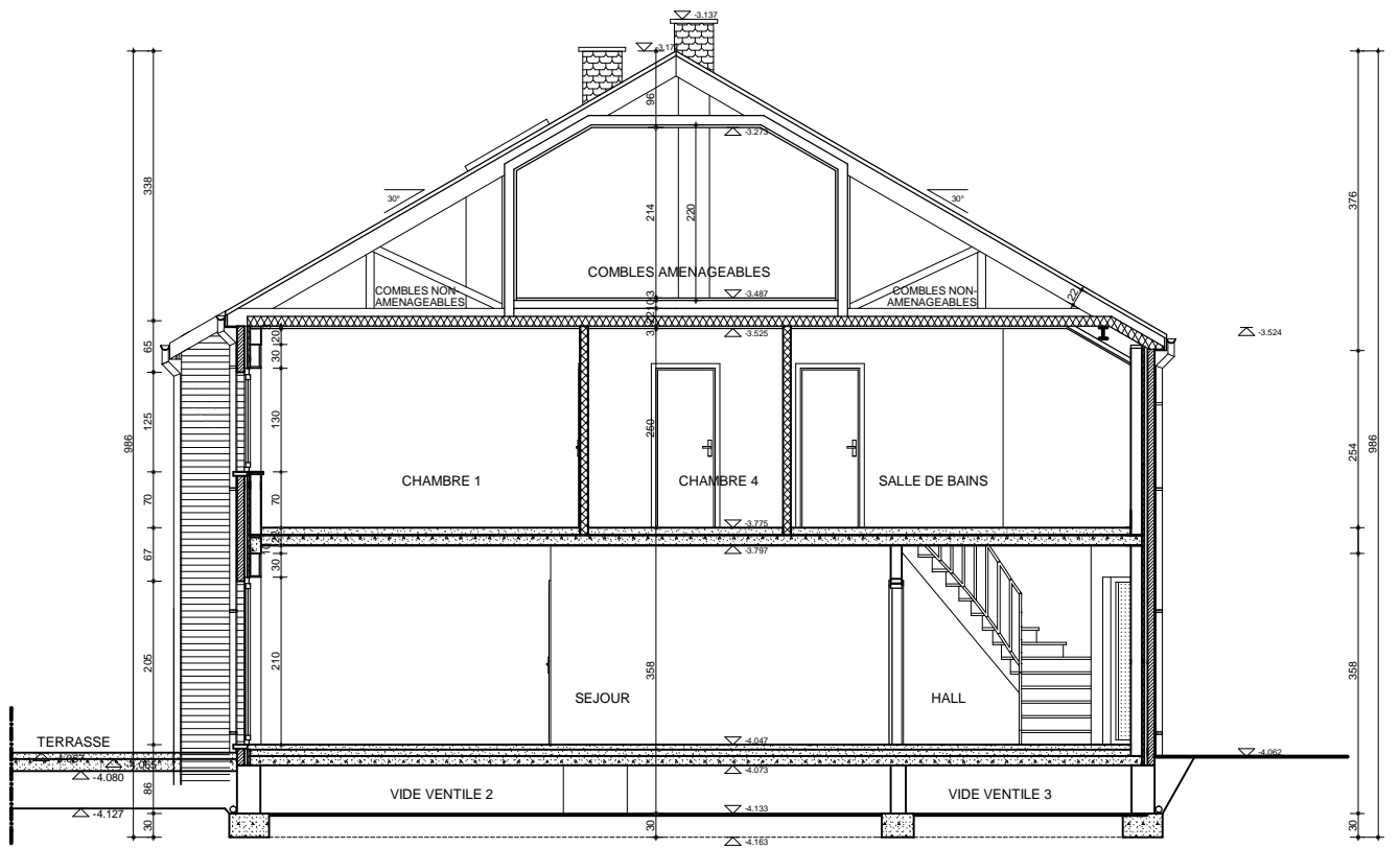
Baelen : Coupe maison 20
