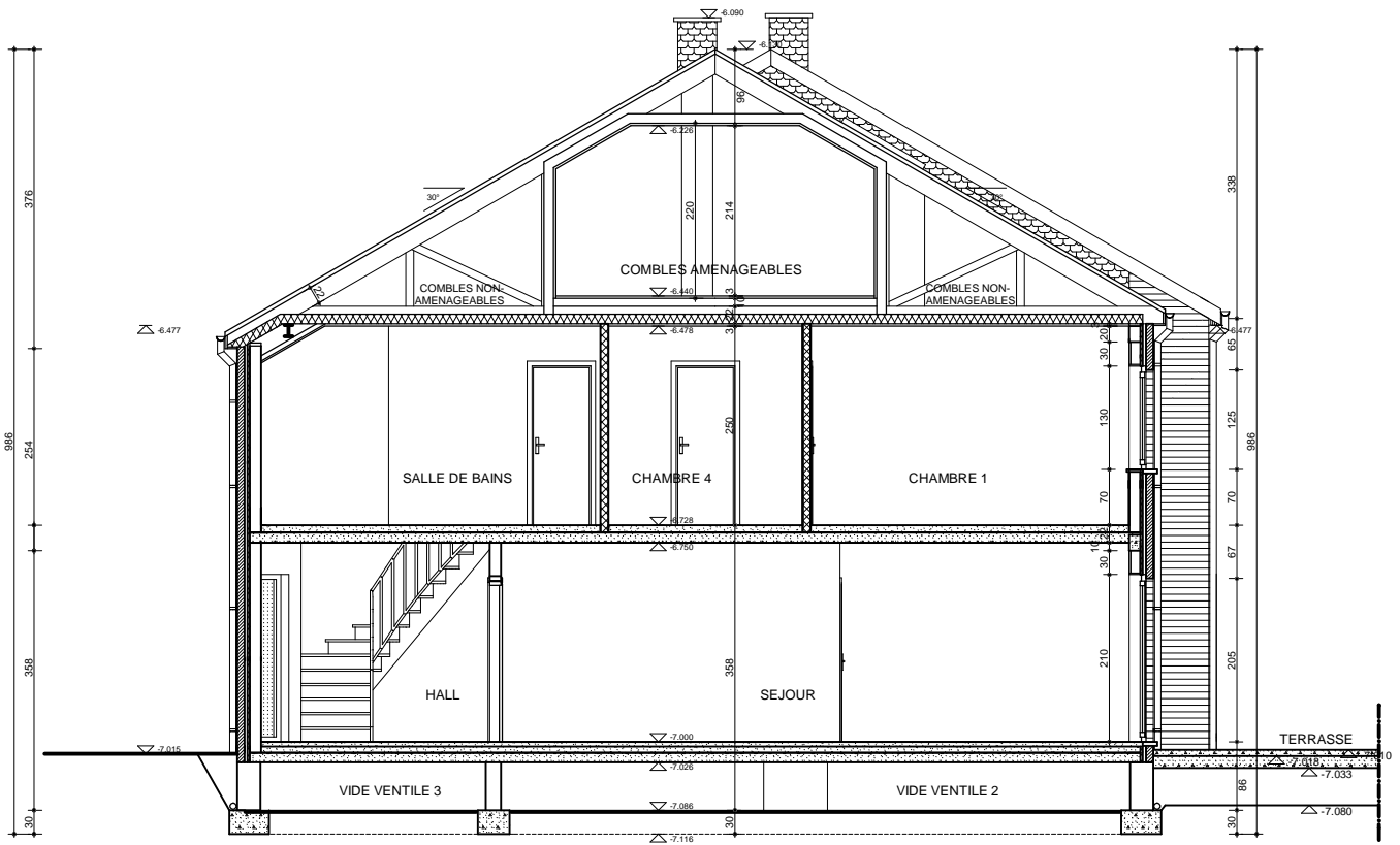
Baelen : Coupe maison 22
