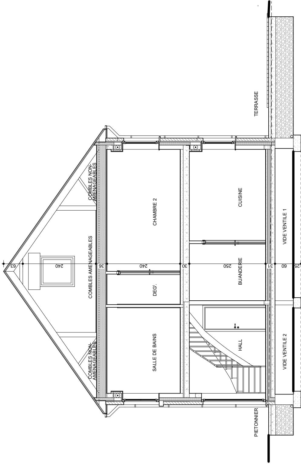
Sainte - Walburge : Coupe A lot 3
