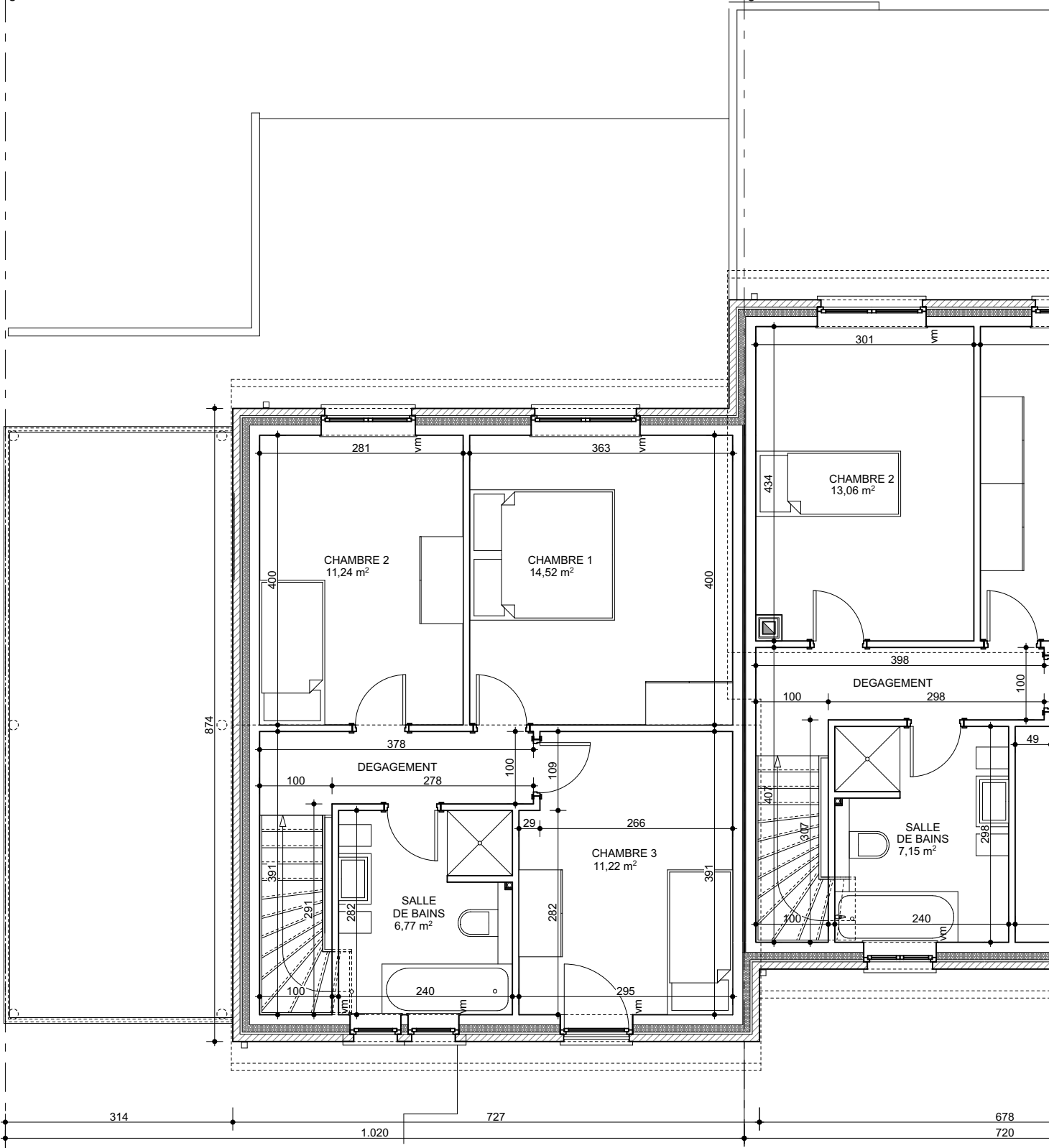
Sainte - Walburge : Etage maison 3
