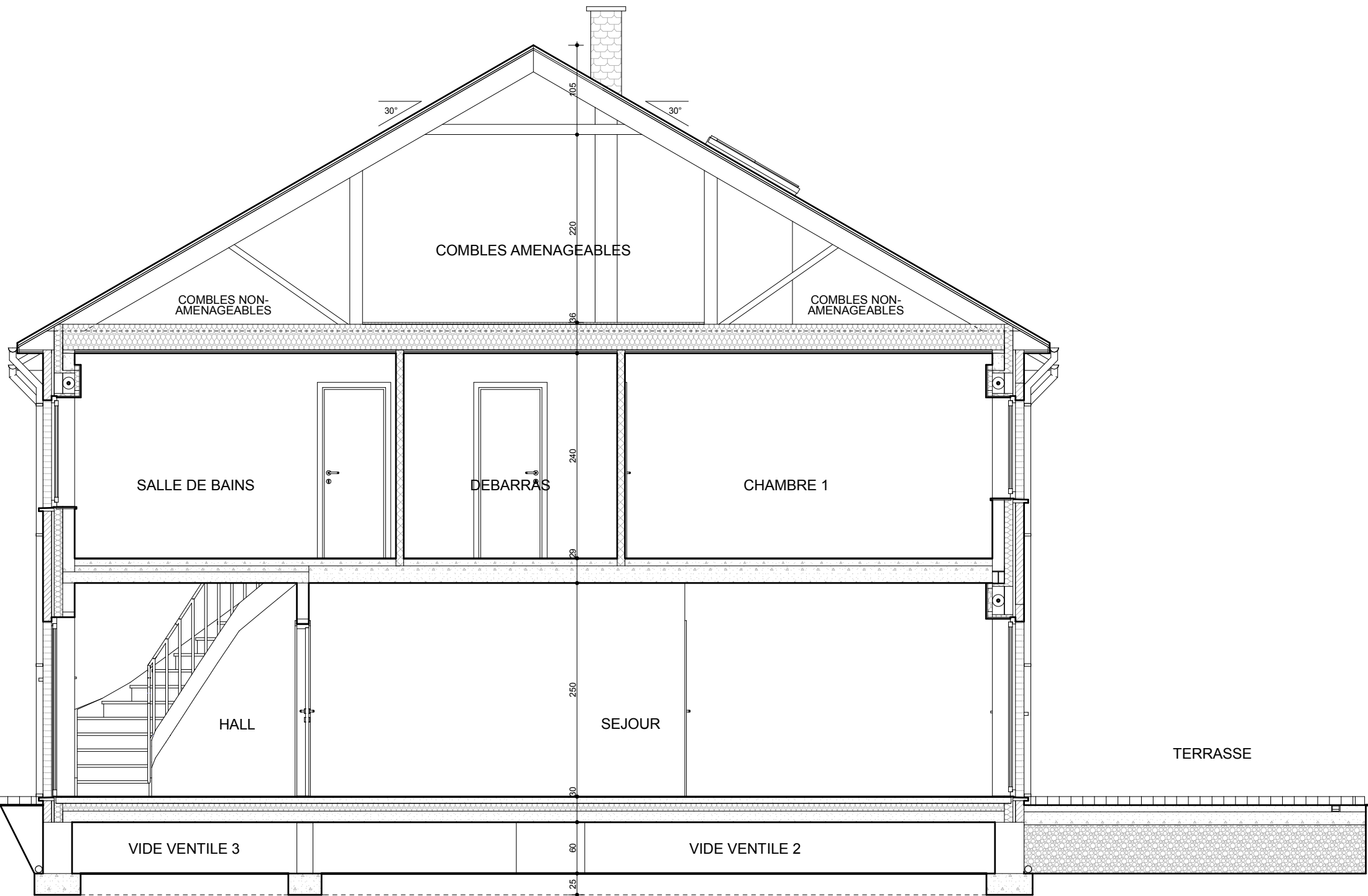
Sainte - Walburge : Coupe BB lot 9
