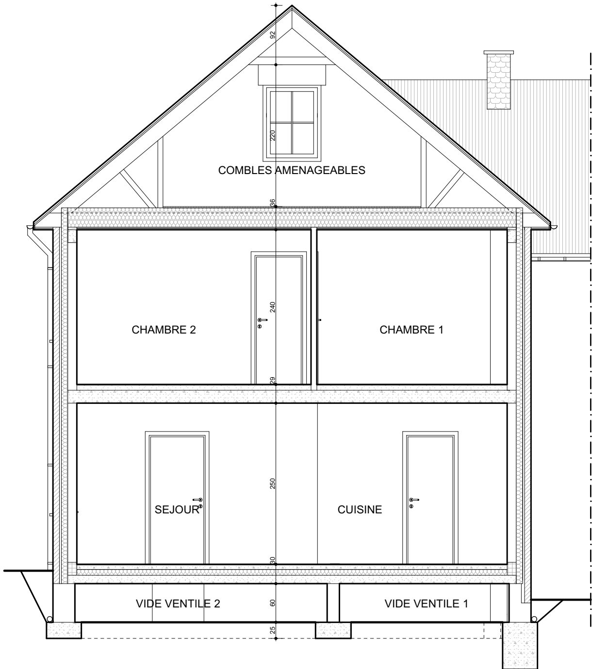
Sainte - Walburge : Coupe CC lot 31
