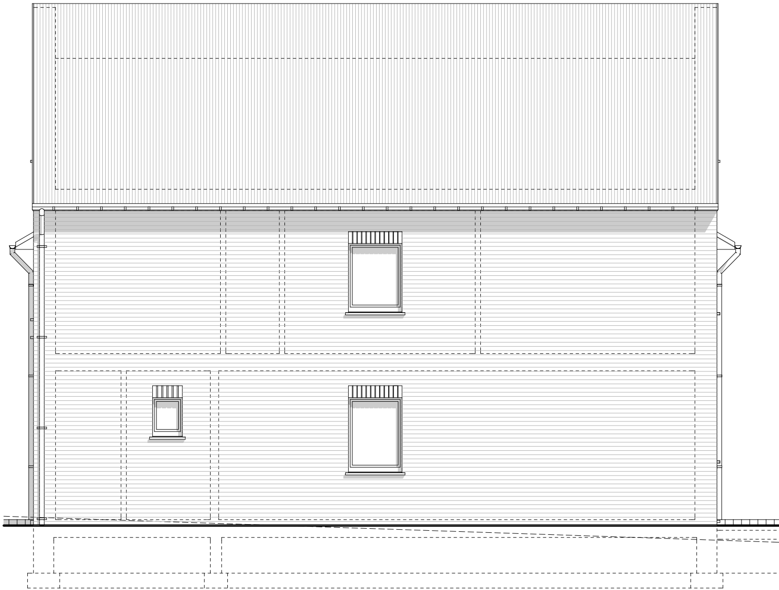
Sainte - Walburge : Façade latérale droite lot 31
