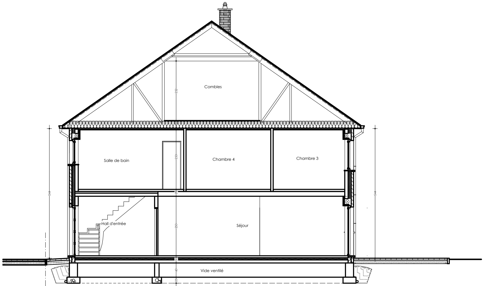
Maison 14 : Coupe BB
