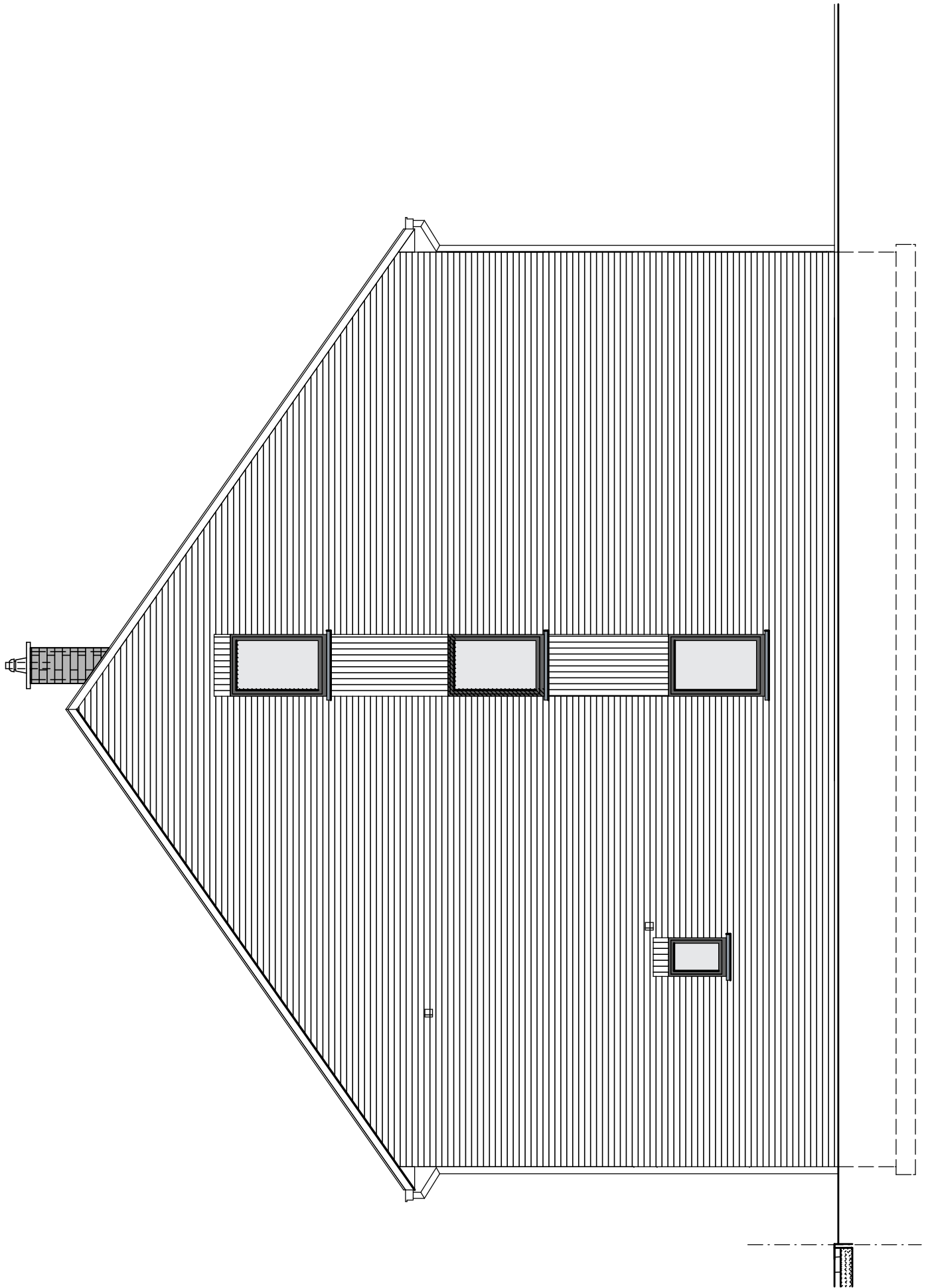
Façade latérale droite : Maison 18
