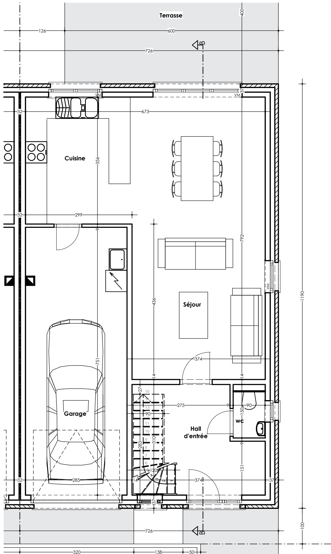
Plan rez-de-chaussée : Maison 18
