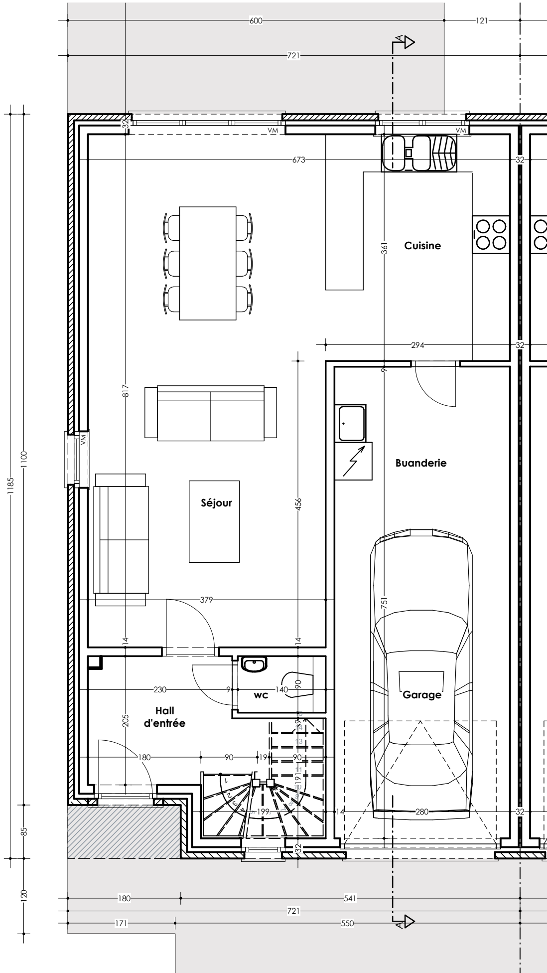
Maison 31 Rez de Chaussée
