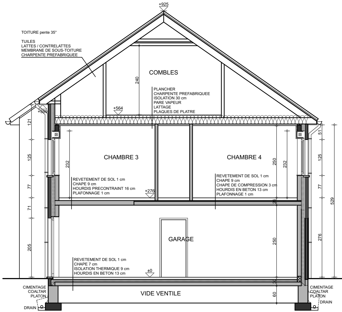
COUPE CC'
