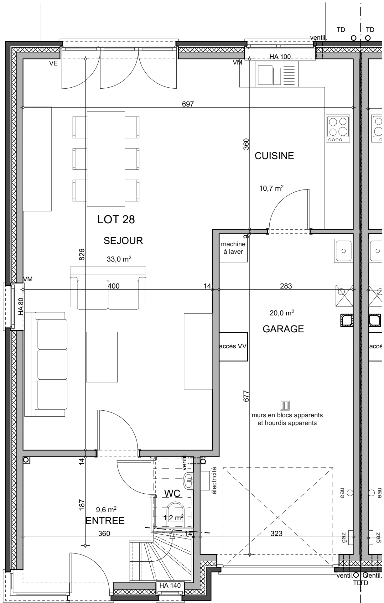
OUPEYE - rue du XI Novembre MAISON 28 - REZ-DE-CHAUSSEE
