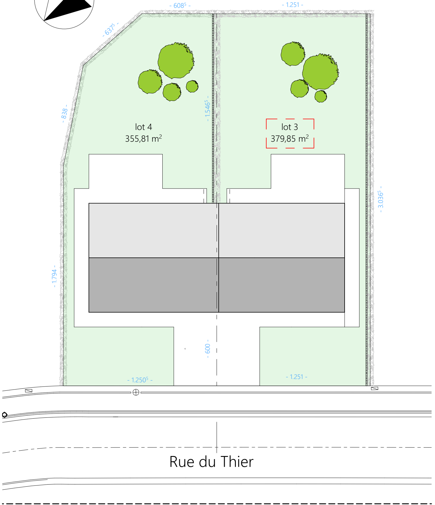
Plan d'implantation
