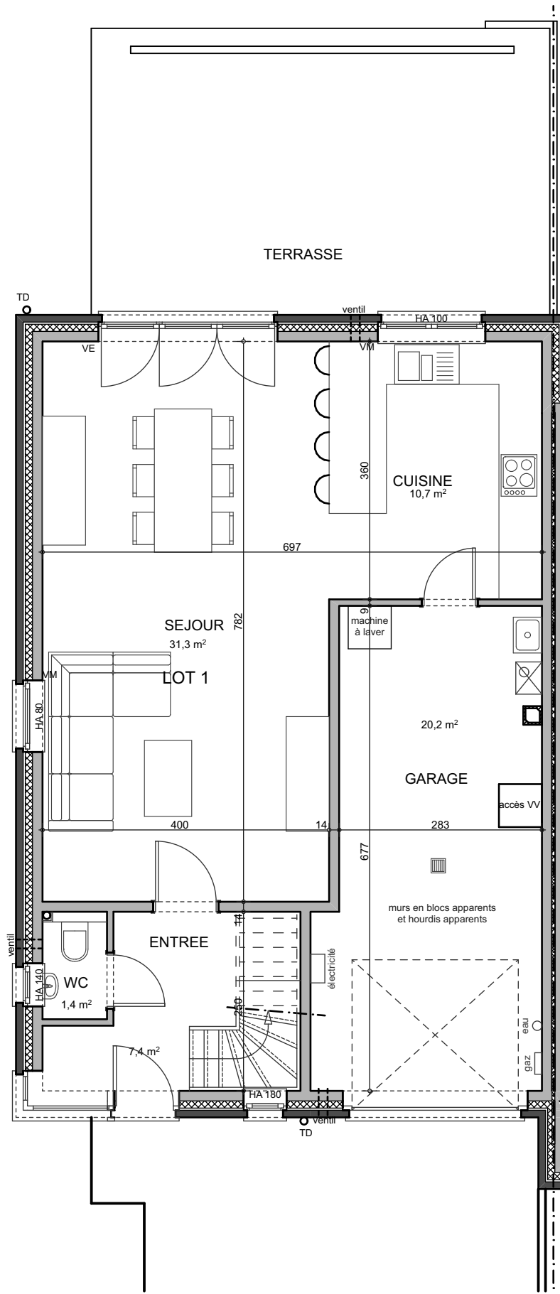
LIERS - CHAUSSEE BRUNEHULT MAISON 1 - REZ-DE-CHAUSSEE
