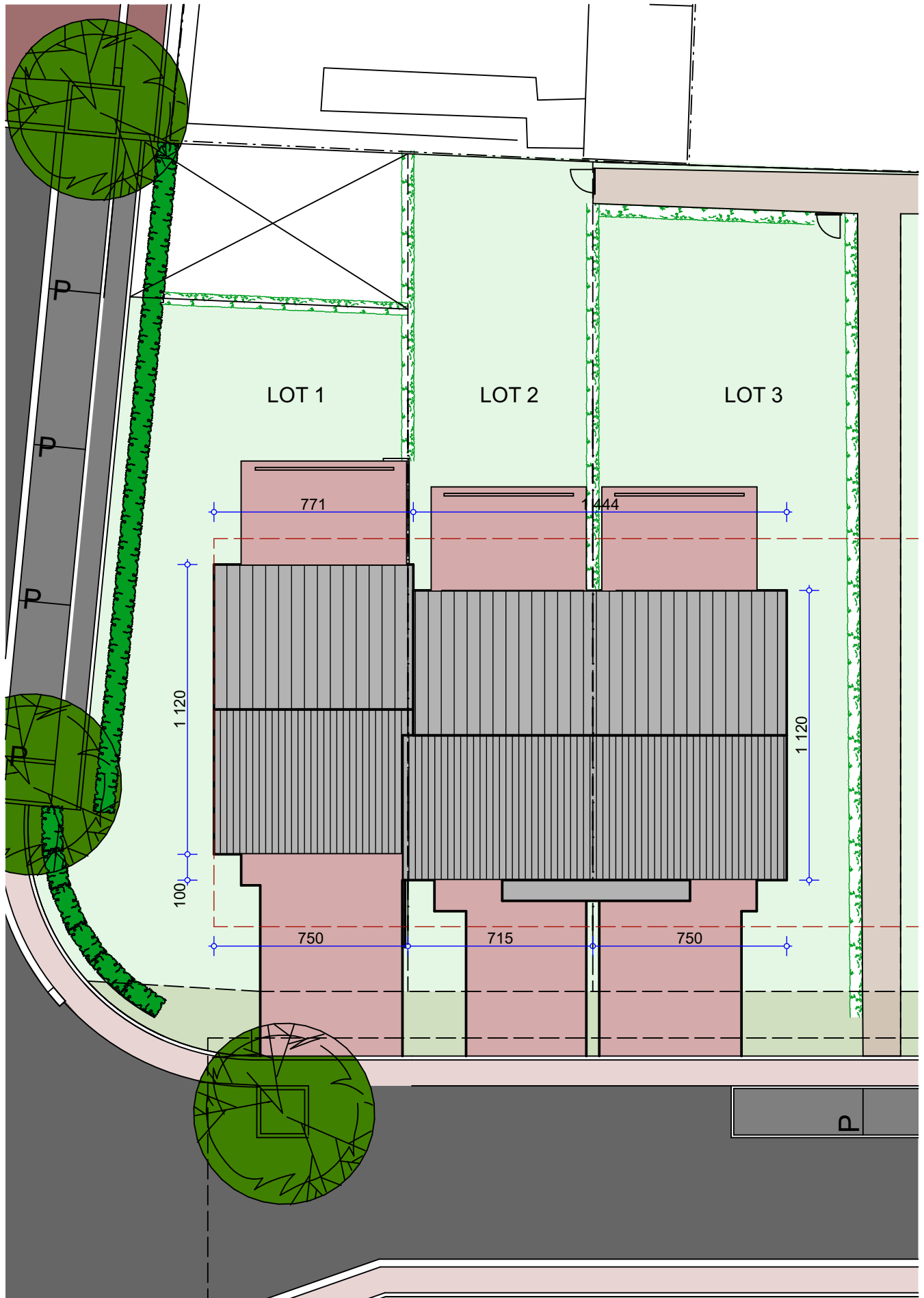
LIERS - CHAUSSEE BRUNEHault MAISON 1 à 3 - IMPLANTATION
