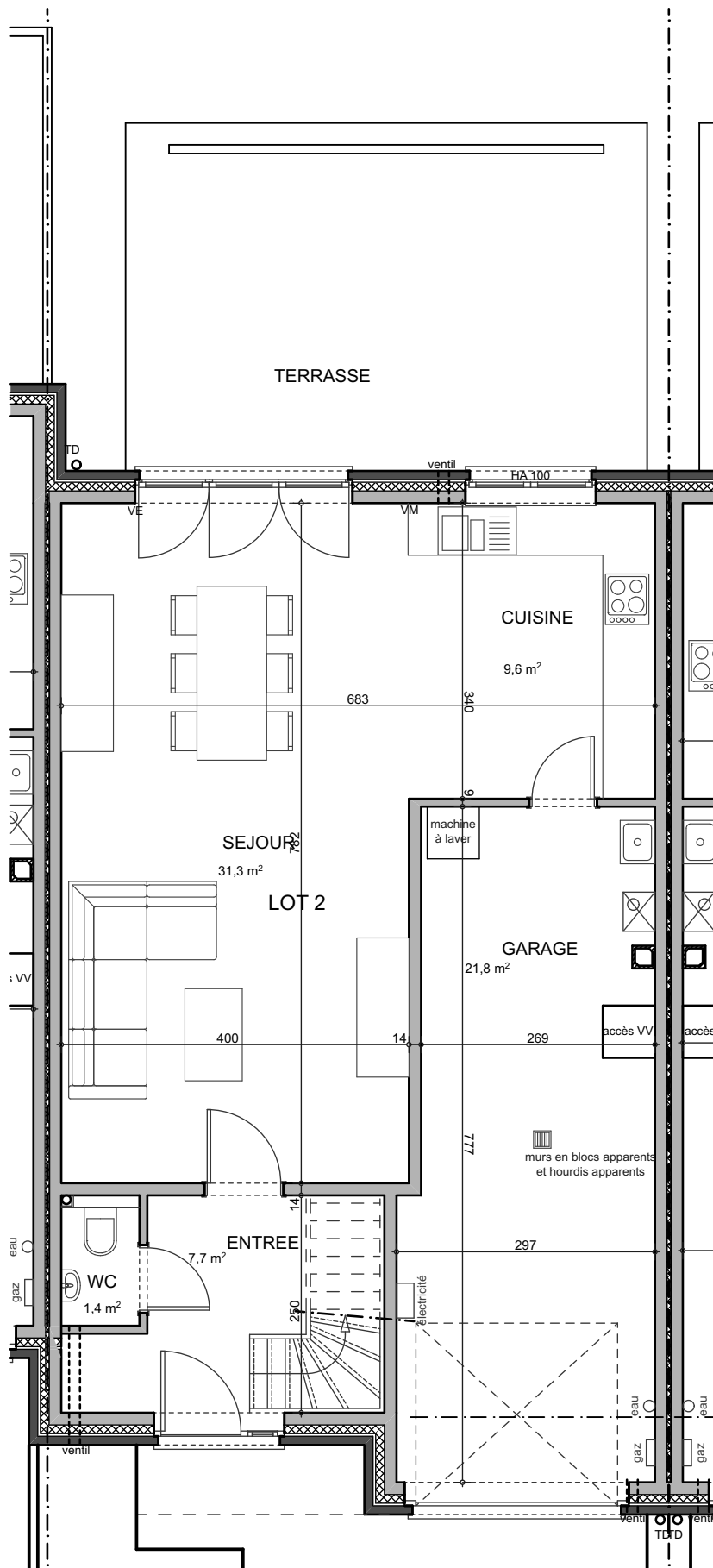
LIERS - CHAUSSEE BRUNEHULT MAISON 2 - REZ-DE-CHAUSSEE
