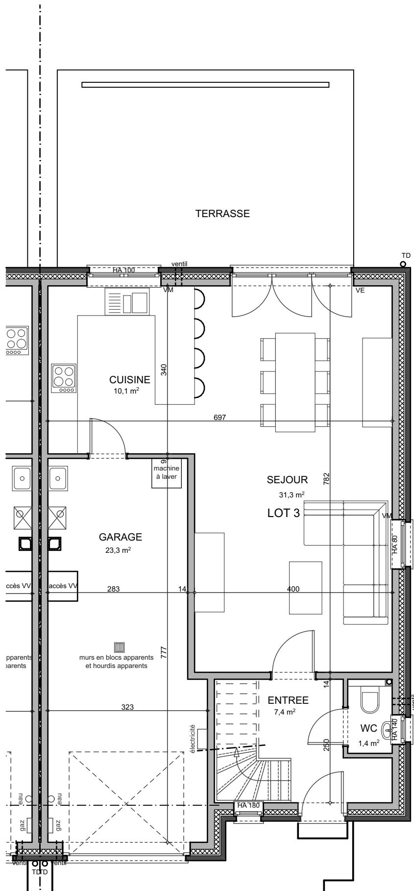
LIERS - CHAUSSEE BRUNEHault MAISON 3 - REZ-DE-CHAUSSEE
