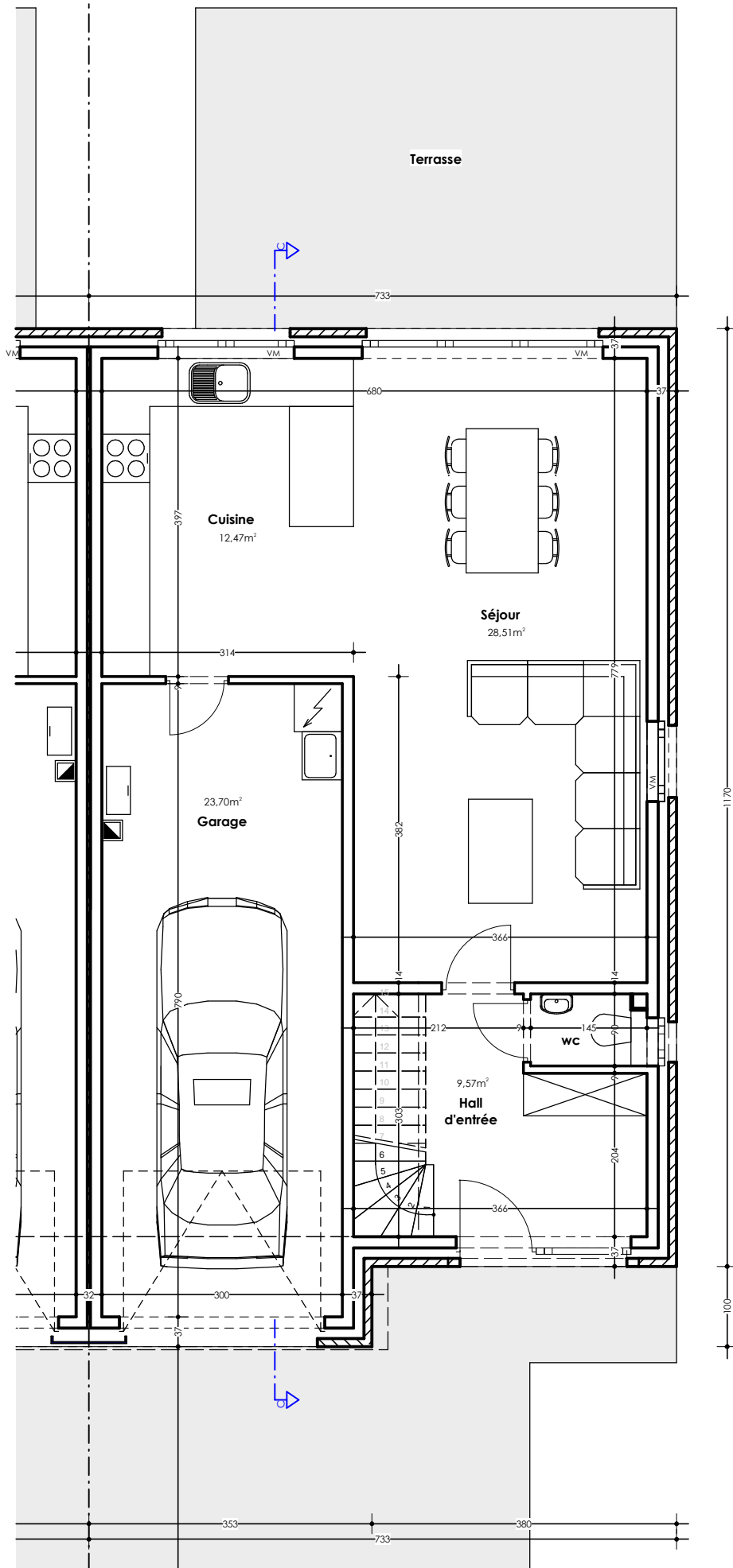
Maison 11 : Plan rez-de-chaussée
