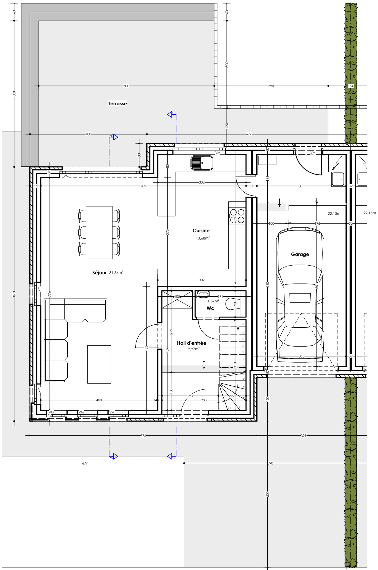
Maison 21 : Plan rez-de-chaussée
