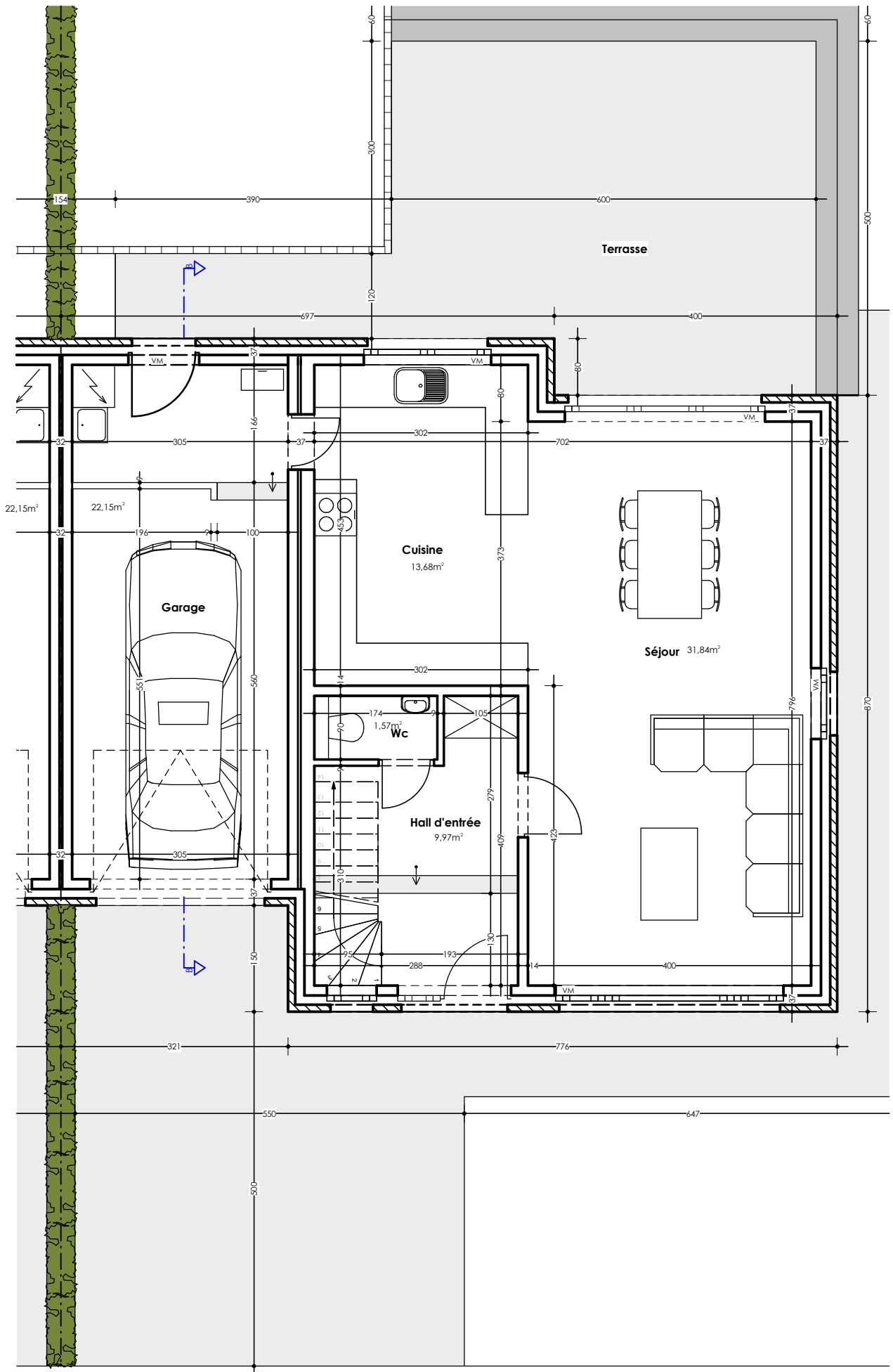
Maison 22 : Plan rez-de-chaussée
