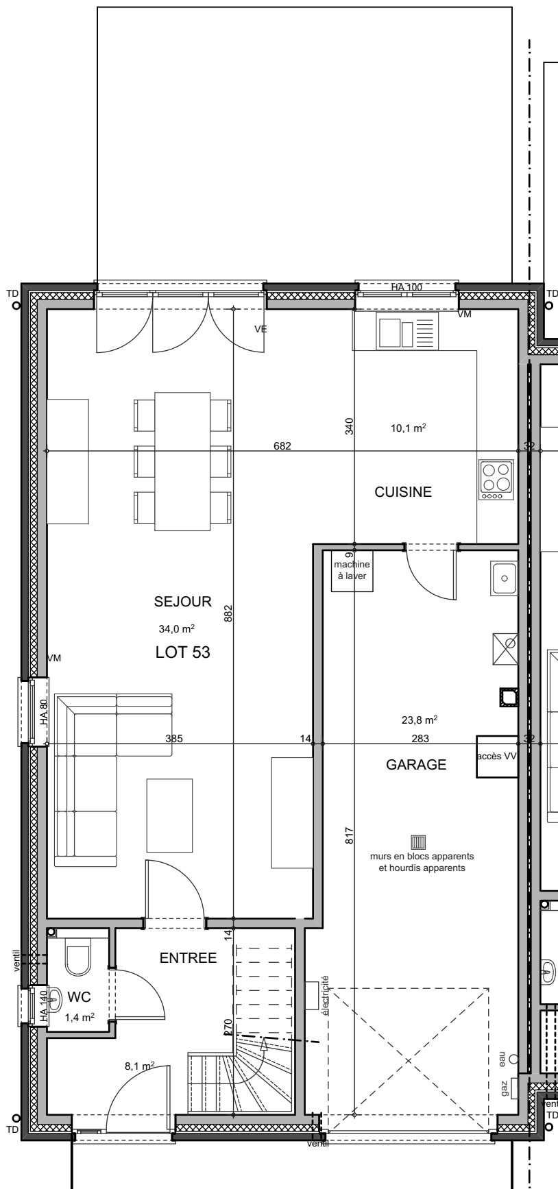
LIERS - CHAUSSEE BRUNEHault MAISON 53 - REZ-DE-CHAUSSEE
