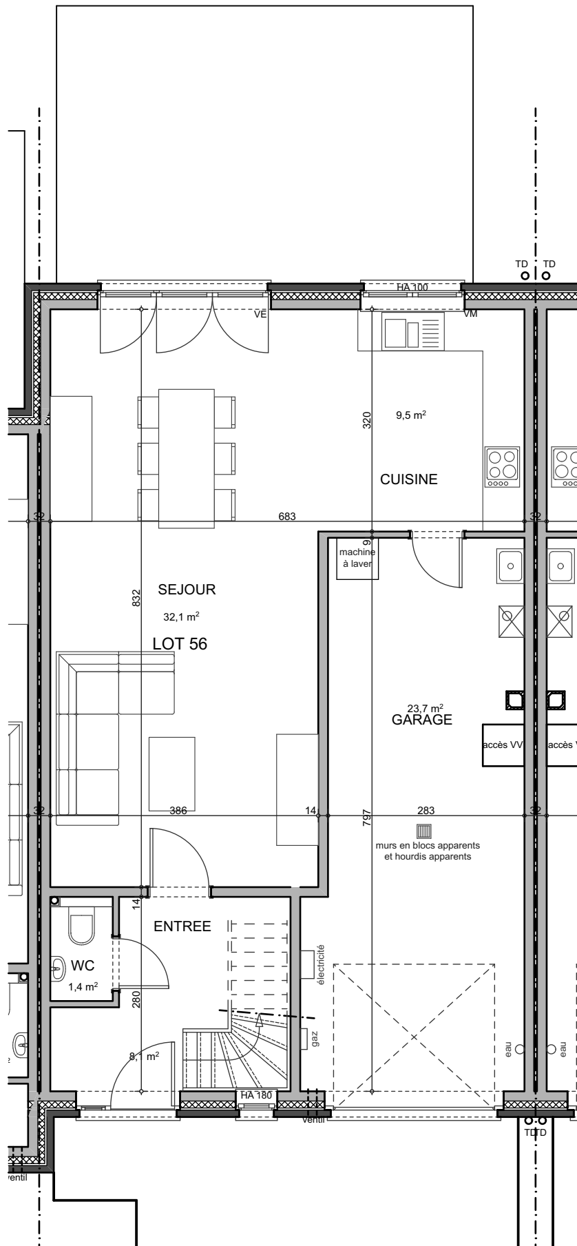
LIERS - CHAUSSEE BRUNEHault MAISON 56 - REZ-DE-CHAUSSEE
