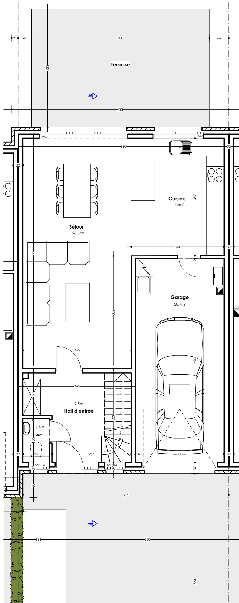
Maison 75 : Plan rez-de-chaussée
