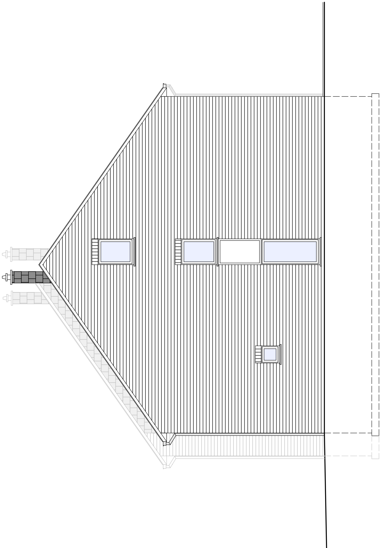
Maison 76 : Façade latérale droite
