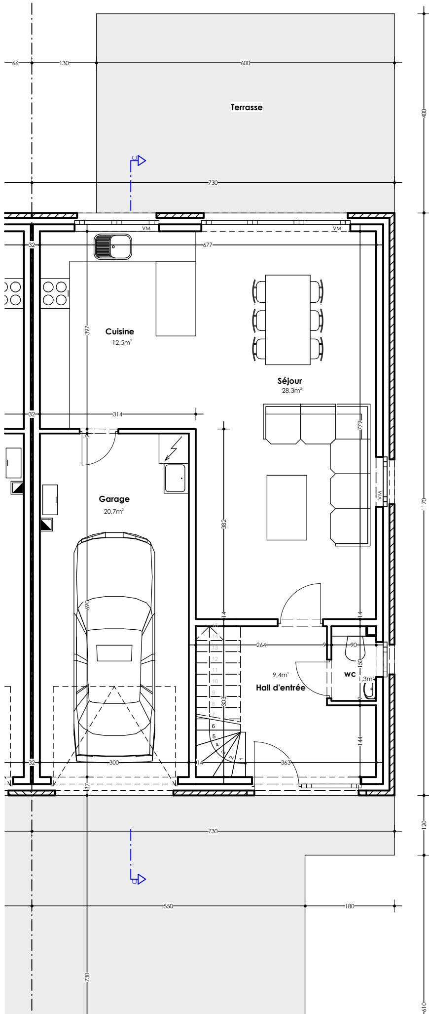
Maison 76 : Plan rez-de-chaussée
