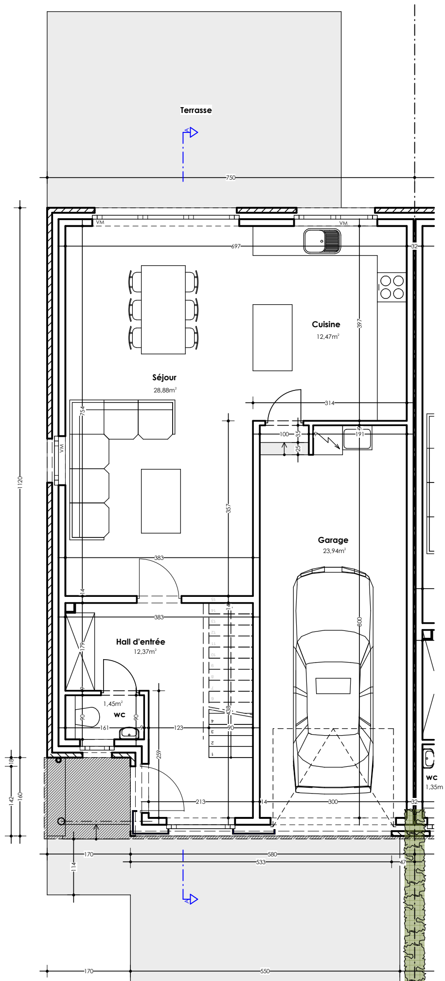
Maison 79 : Plan rez-de-chaussée
