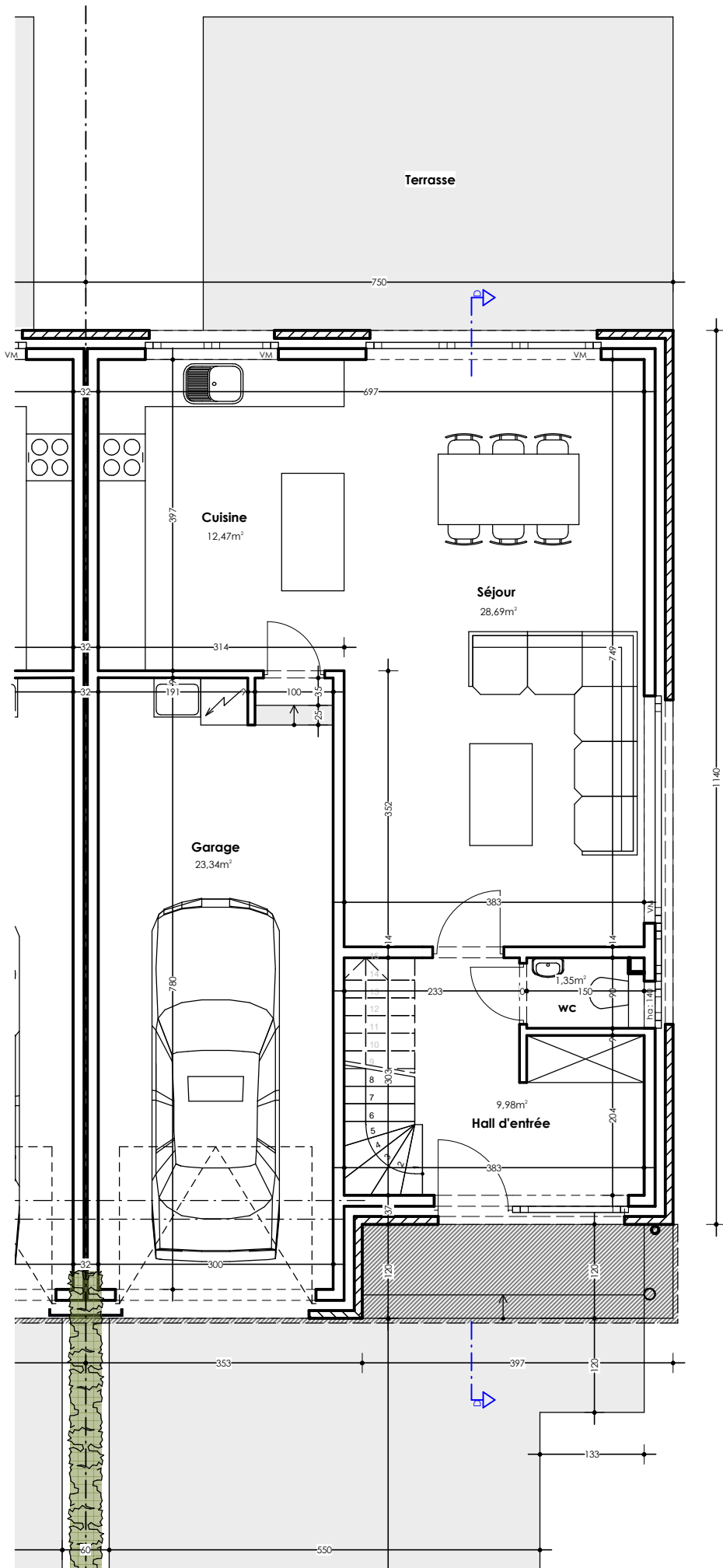
Maison 82 : Plan rez-de-chaussée
