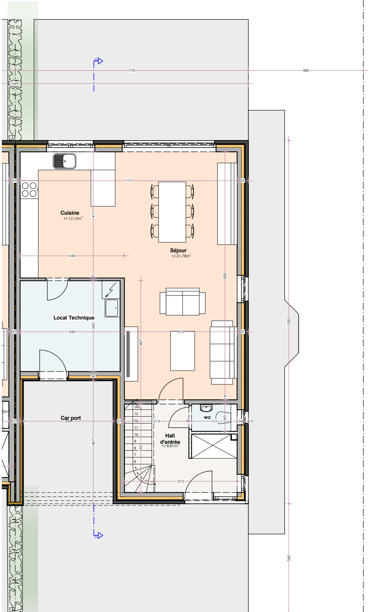
Maison 16 : Plan rez-de-chaussée
