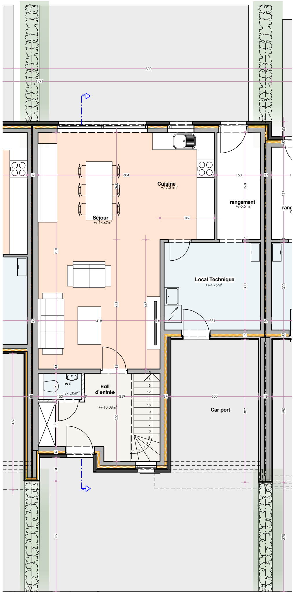
Maison 18 : Plan rez-de-chaussée
